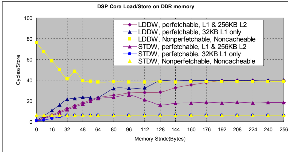
图 6 DSP 核对于 DDR Load/Store 的时延
