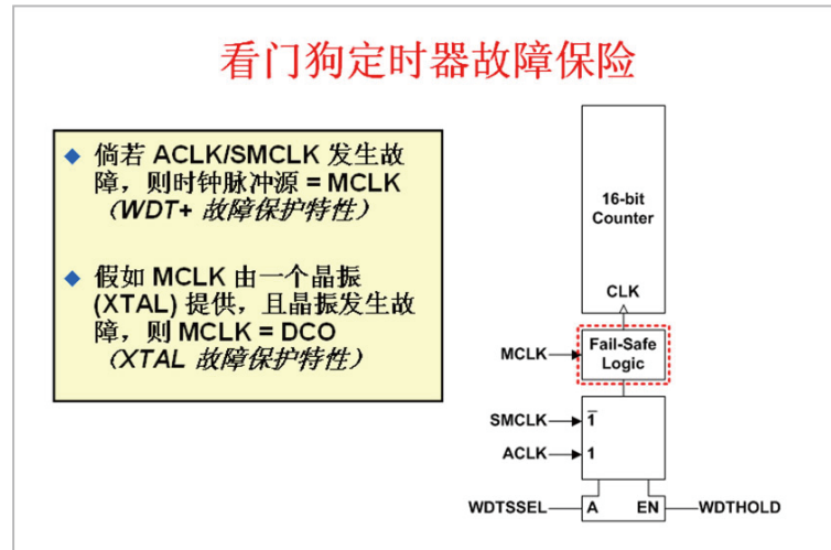
图5.8画出了看门狗定时器故障保护的运作方式。
