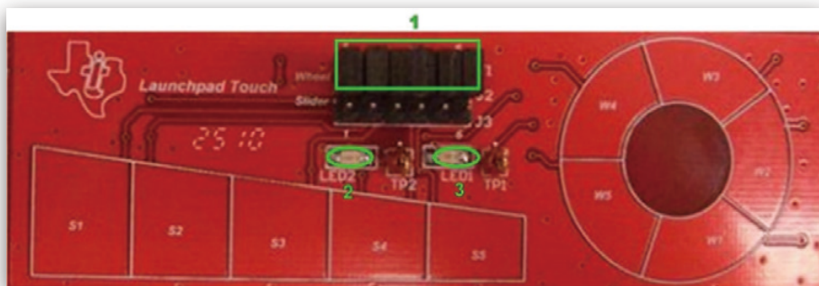
图4. 触摸感应子卡设置示意图
