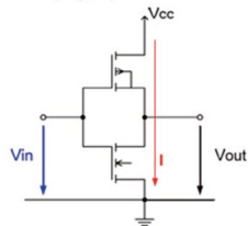
(Digital) CMOS Inverter
