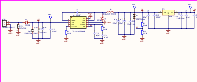
电源电路
