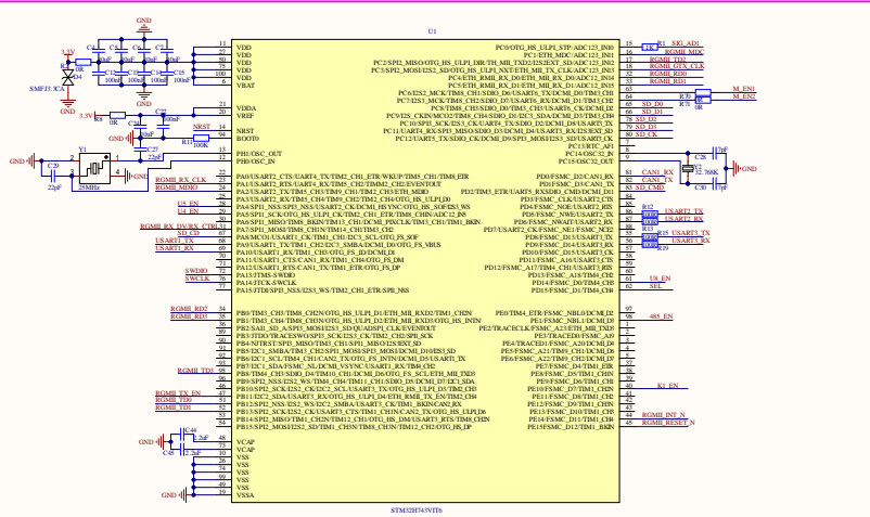
MCU电路
