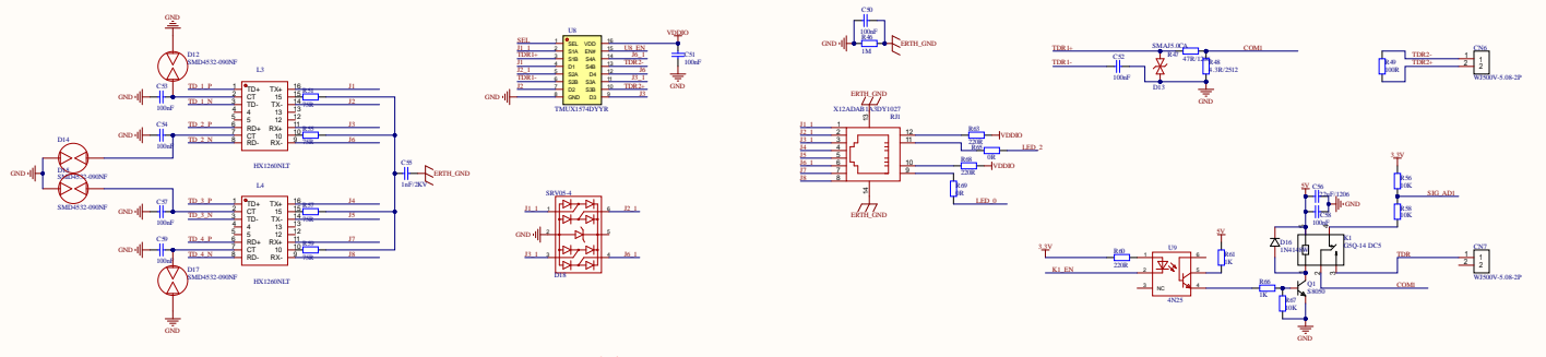
TDR网卡电路
