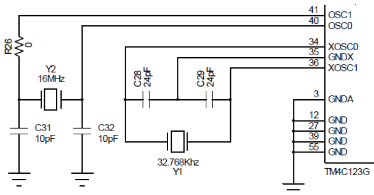
时钟电路
