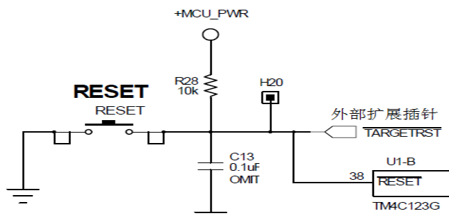
复位电路
