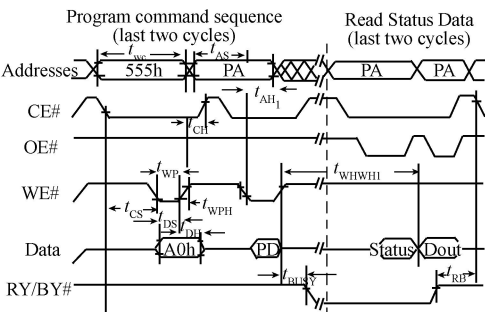
图 4 AM29LV800 写操作时序图
