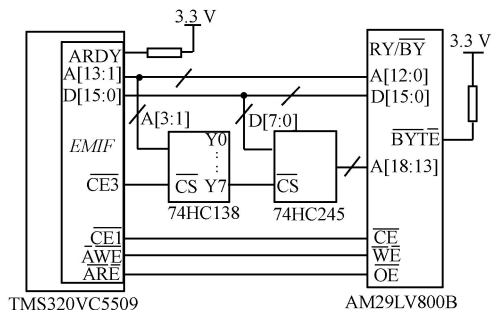
图 2 TMS320VC5509 与 AM29LV800 的硬件连接示意图
