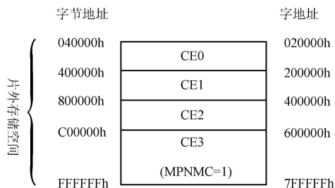
图 1 外部存储空间的划分
