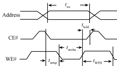
图 3 TMS320VC5509 中三个时间的定义
