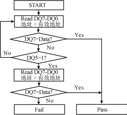
图 5 Data # polling 位的算法
