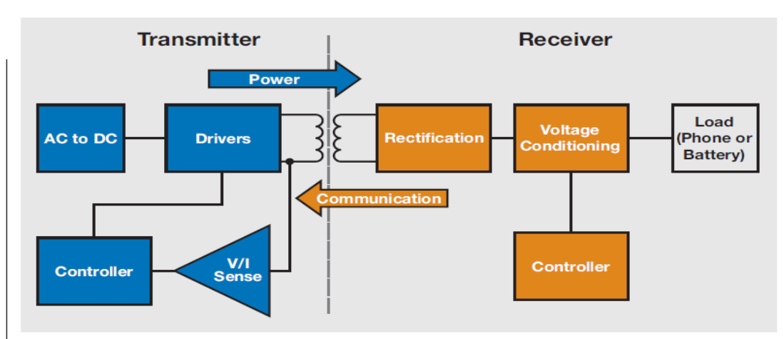
图 1 典型无线充电功能结构图
