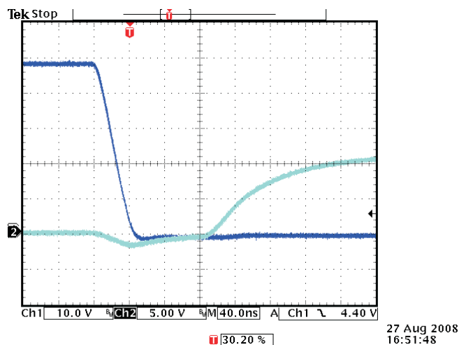
Figure 5. Q4 (CD Leg) at 5.5-A Load
