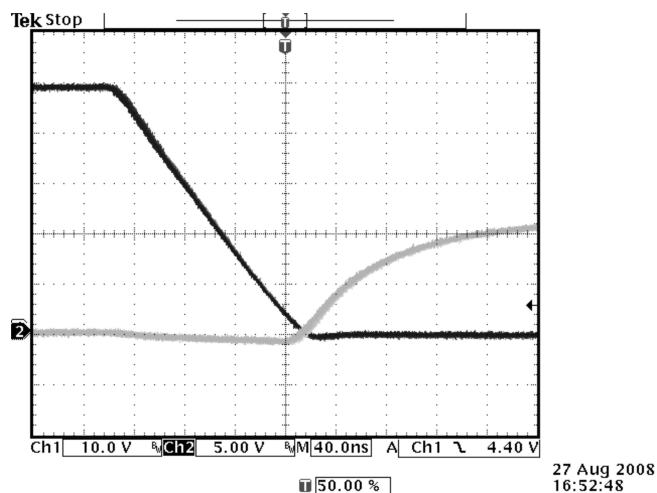
Figure 7. Q4 (CD Leg) at 0-A Load
