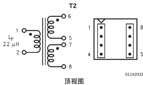
图16：Coilcraft Q4337-B
