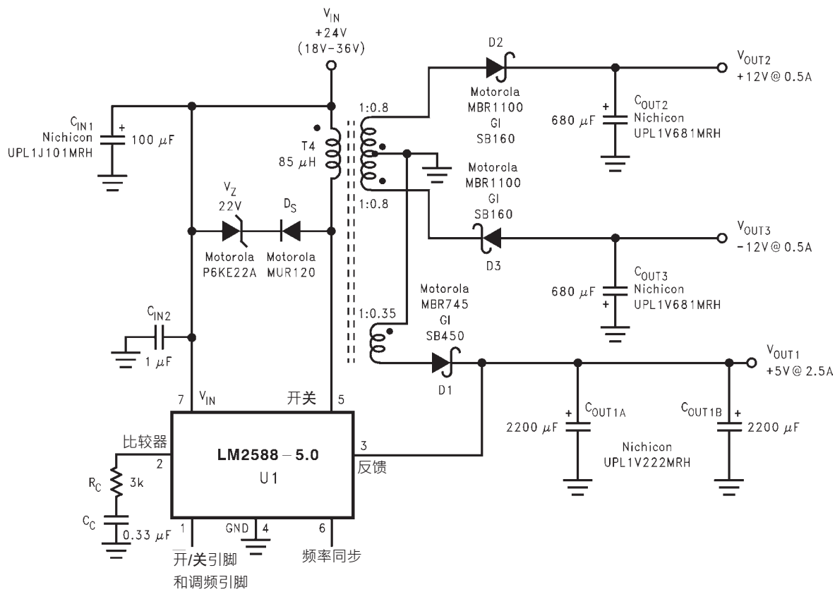
图12. 三路输出回扫式稳压器
