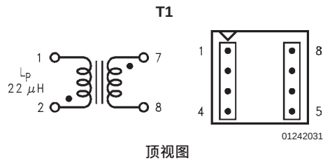
图15：Coilcraft Q4434-B
