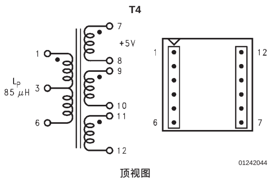
图28. Renco RL-5535
