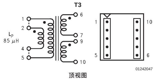
图31. Schott 67140920
