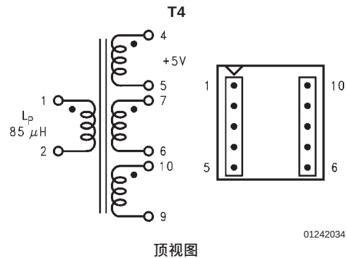
图18：Coilcraft Q4344-B
