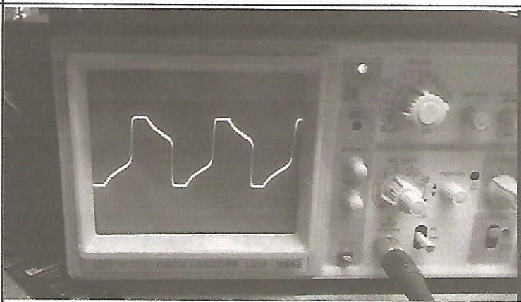
正常波形图
