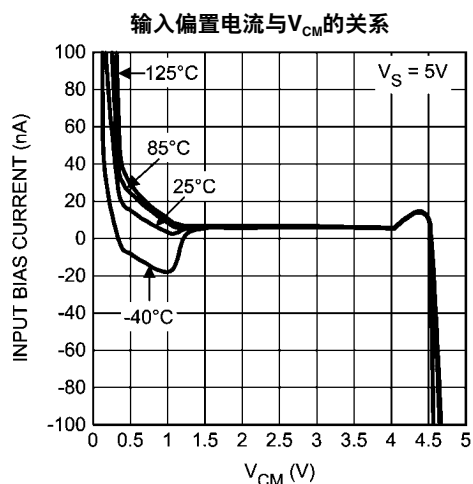
图3. LMP7731的输入偏置电流与 V_{CM} 的关系 (典型特征)
