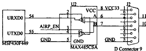
图3 MSP430F449 与 PT220 的接口电路
