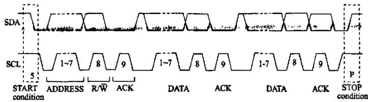
图7 I 2 C总线的读写时序
