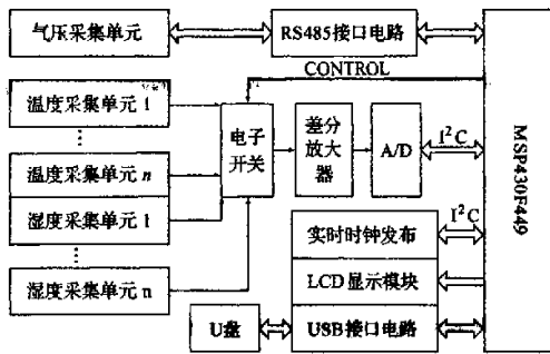
图1 气象数据采集系统框图
