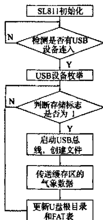
图8 SL811实现U盘数据存储的流程图
