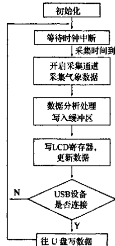
图6 系统主程序流程图
