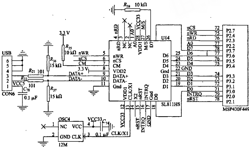
图5 MSP430F449与SL811的USB接口电路
