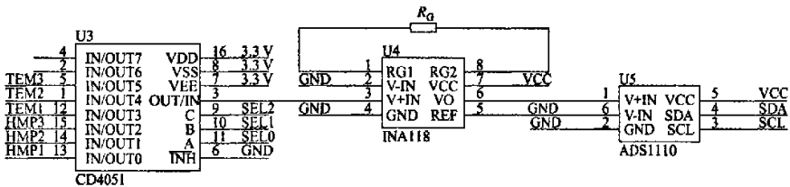
图2 温湿度信号采集电路
