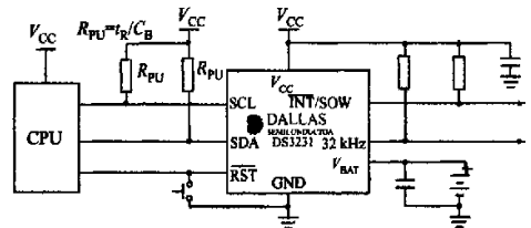
图4 DS3231 的典型工作电路图
