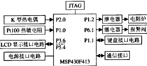
图 2 温度控制硬件框图
