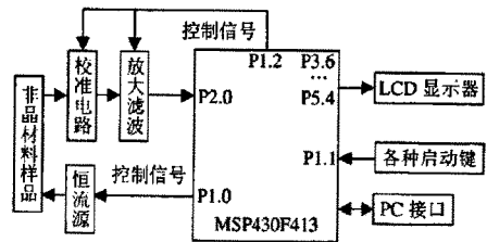
(b) 电阻率测试系统硬件框图
