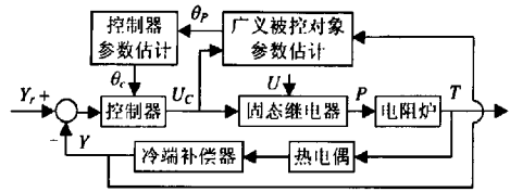
图 3 电阻炉温控系统
