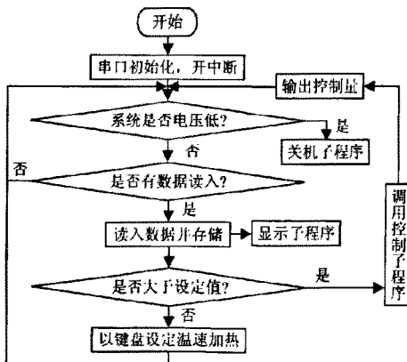
图 5 温控系统主程序流程图
