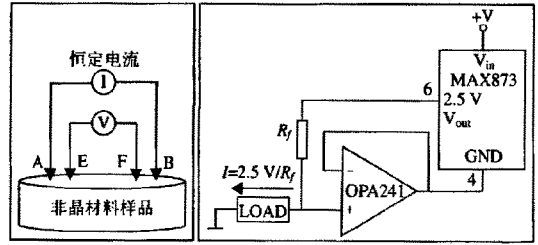
(a) 四探针测试及恒流源电路
