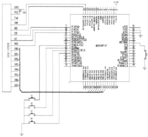
图1 实验原理图
