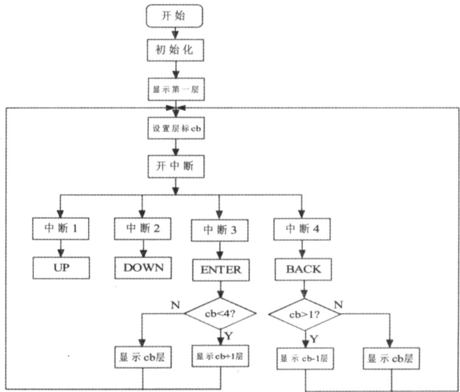
图 3 程序流程图
