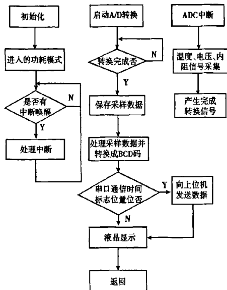
图7 程序流程图
