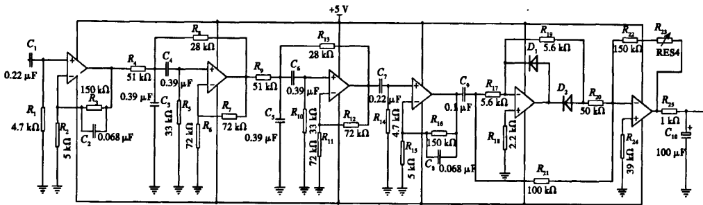
图 3 电池内阻检测电路
