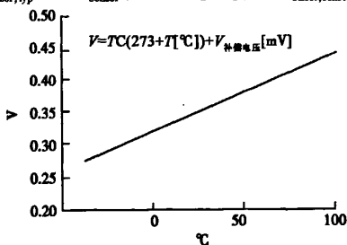
图 5 温度特性曲线
