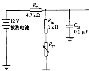
图 4 电压检测电路
