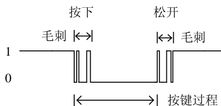
图 2.2.2 按键过程产生的毛刺
