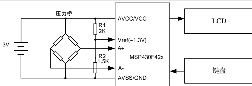
图 2.7.3 用比值测量法消除激励电压变化对压力测量的影响
