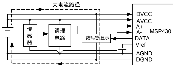
图 2.7.18 合理的接地
