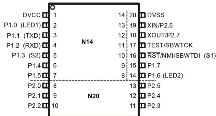
图 5. 器件引脚分配
