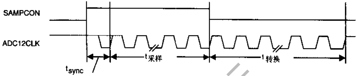
图 15.17 脉冲采样模式时序
