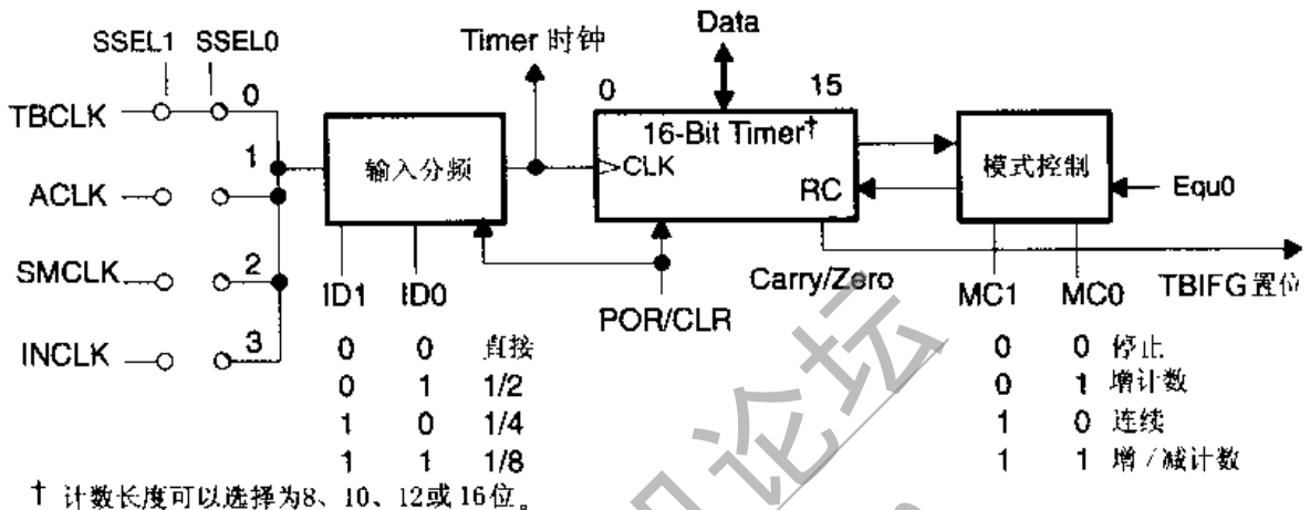
图 11.3 16 位定时器结构
