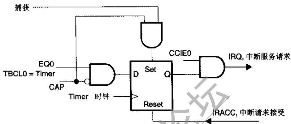
图 11.27 CCR0 中断标志
