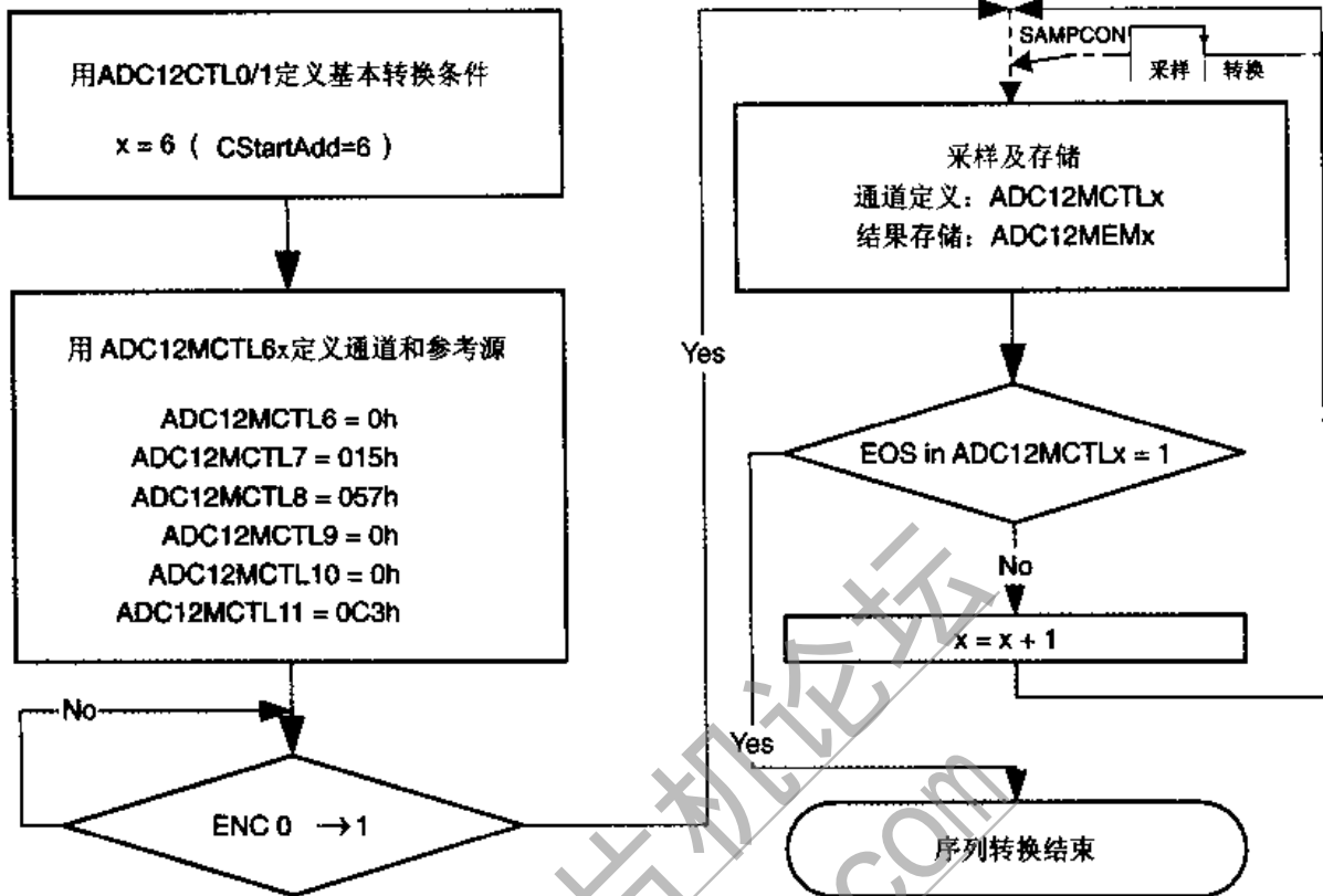
图 15.9 序列转换模式的流程
