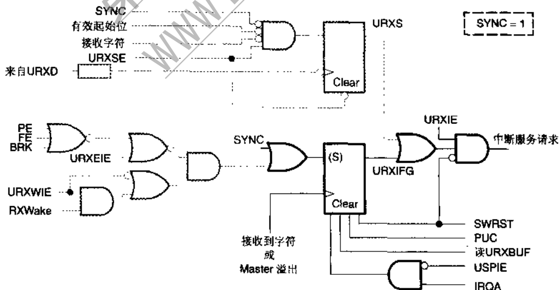
图 13.11 接收中断条件
