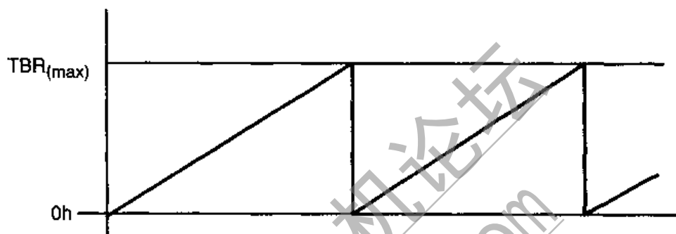
图 11.9 连续模式
