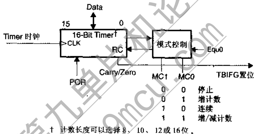
图 11.2 模式控制
