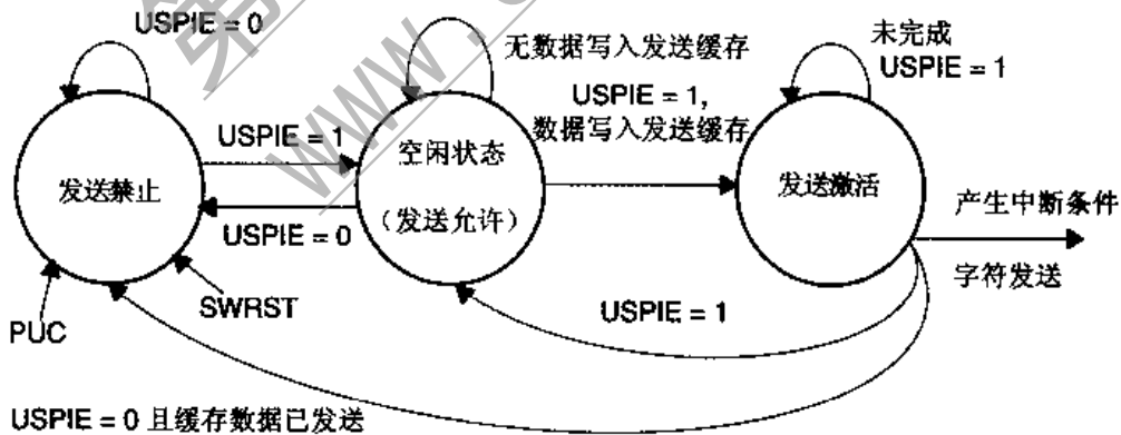
图 13.9 MSP430 为主机的发送允许状态图
