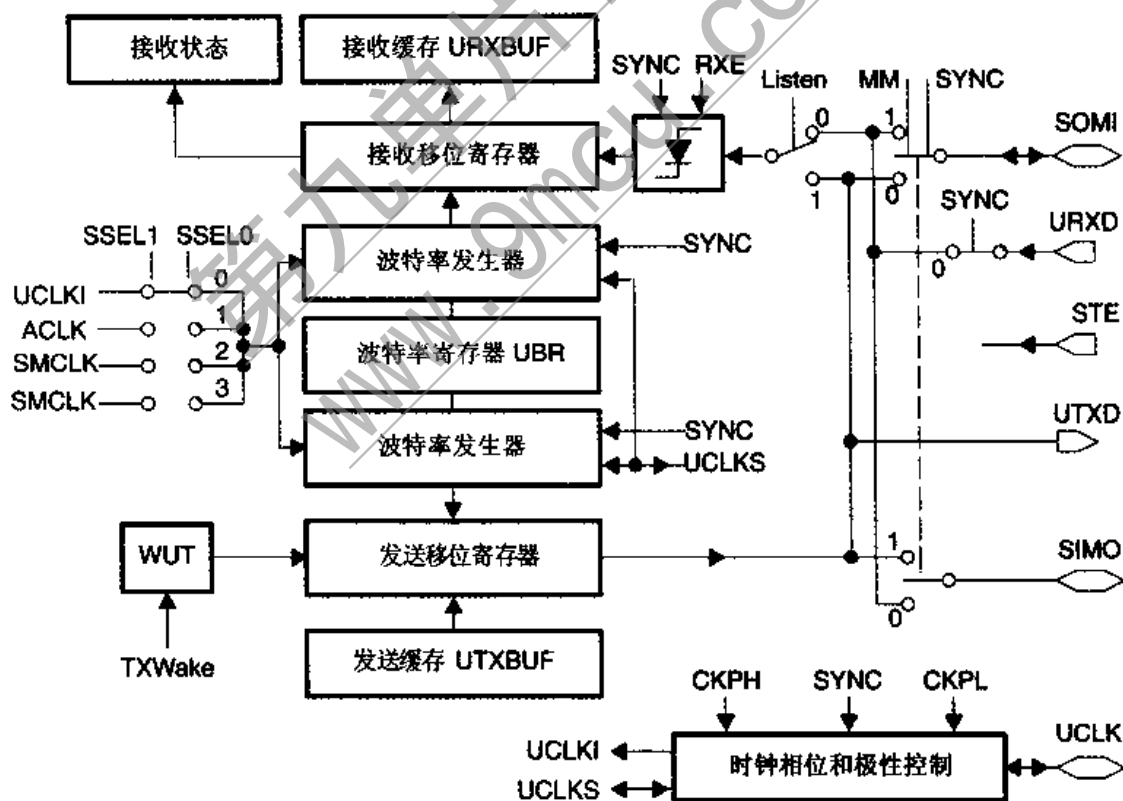
图 12.1 USART 功能框图
