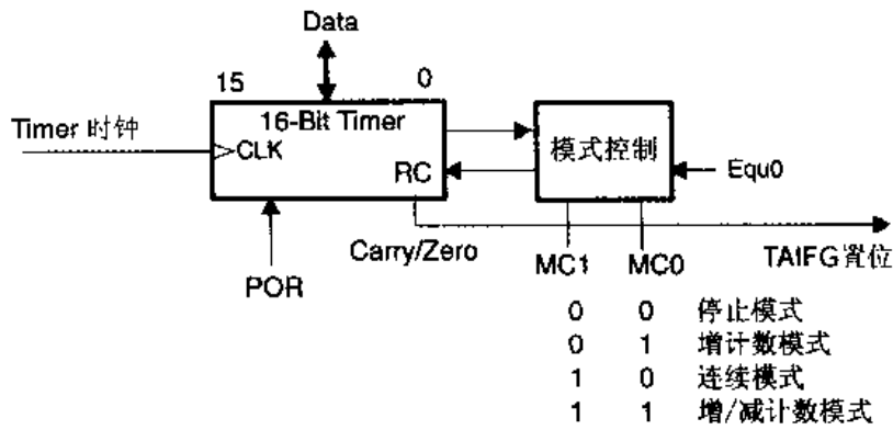
图 10.2 模式控制
