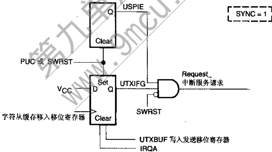
图 13.13 发送中断操作
