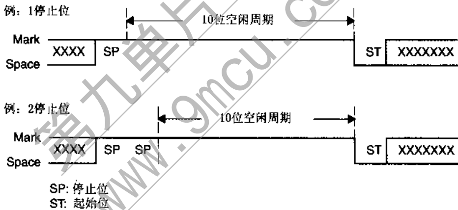
图 12.8 USART 接收空闲检测
