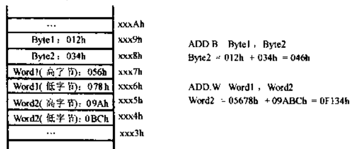
图 4.5 字和字节操作
