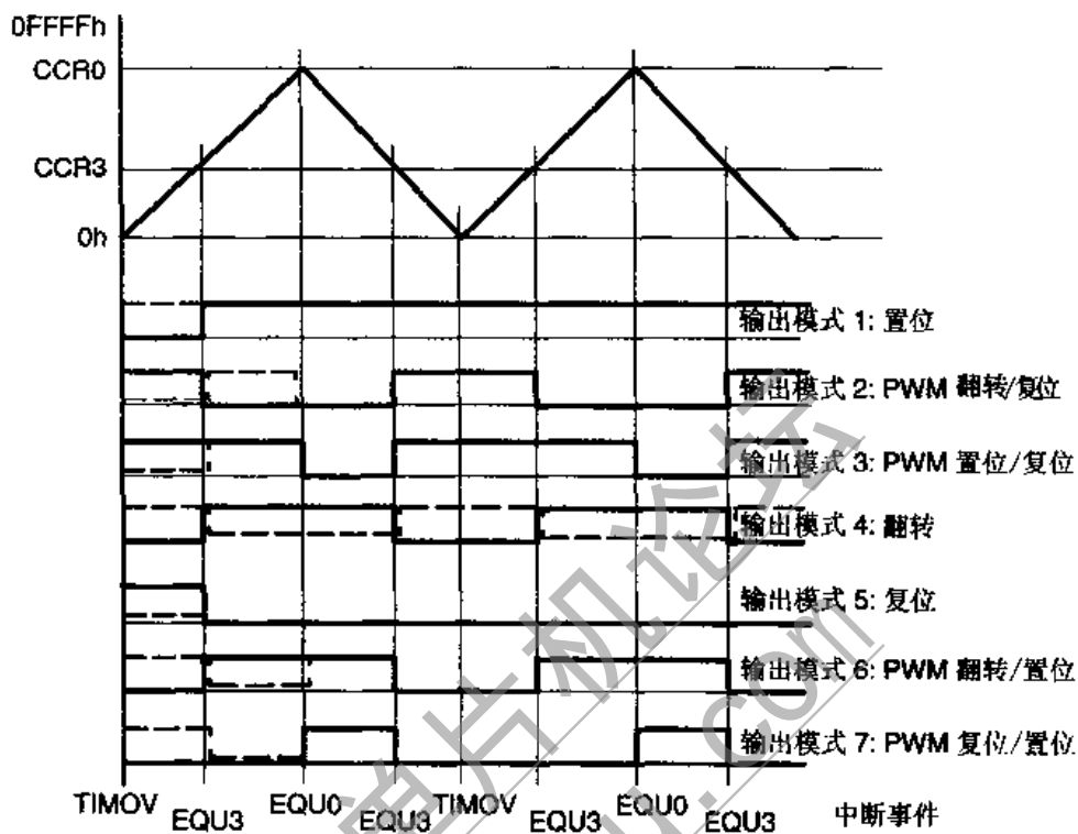
图 10.26 增/减计数模式实例
