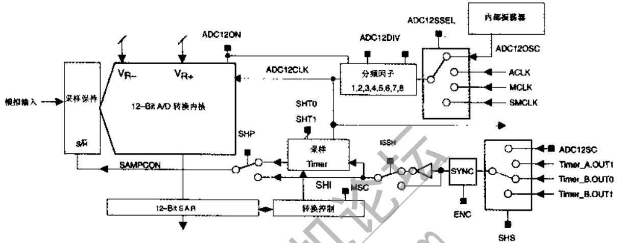
图 15.14 ADC12 中的采样/保持电路
