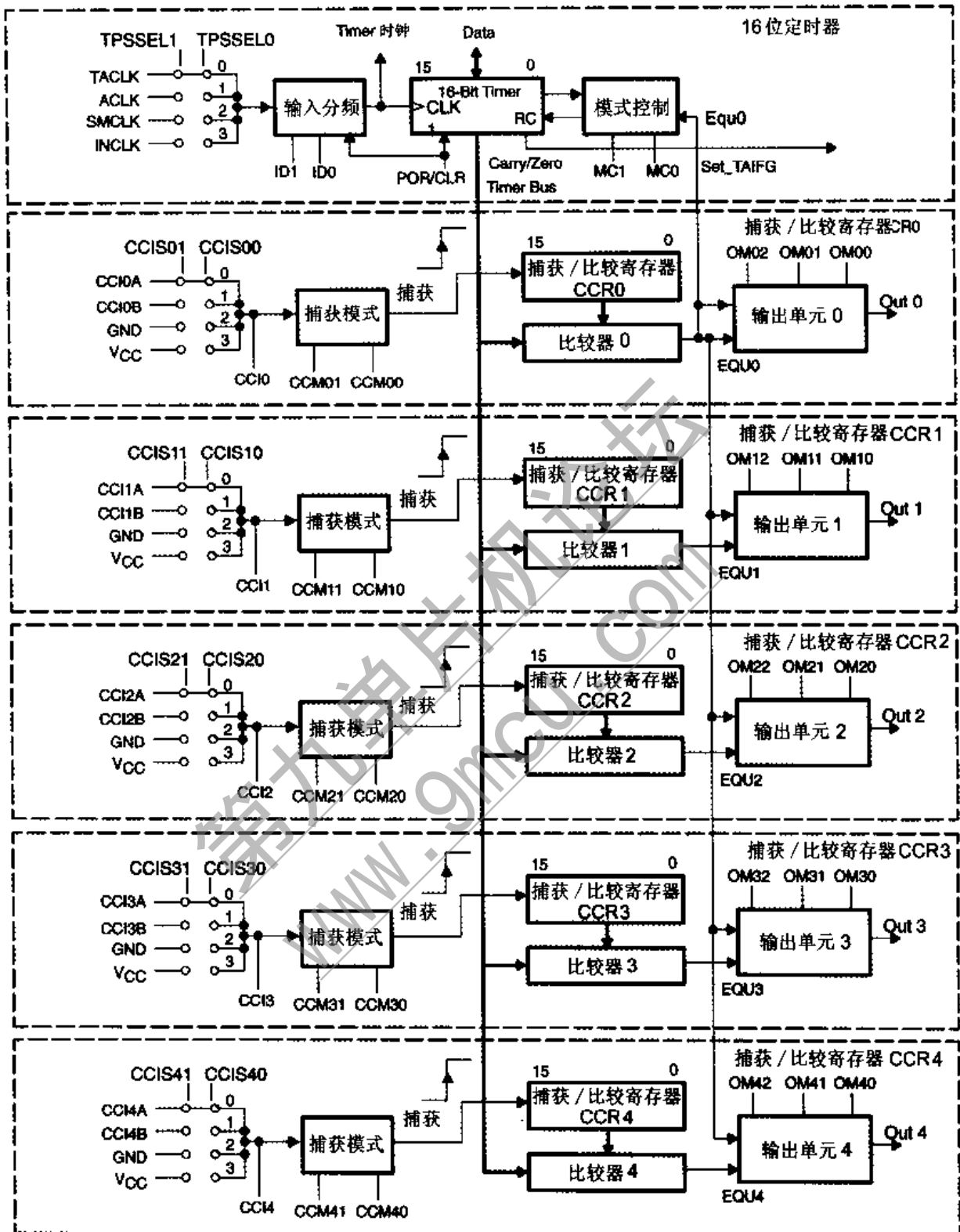
图 10.1 Timer_A 结构
