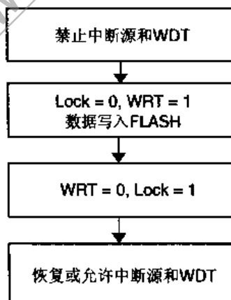
图 4.18 同一模块编程一个字的程序流程
