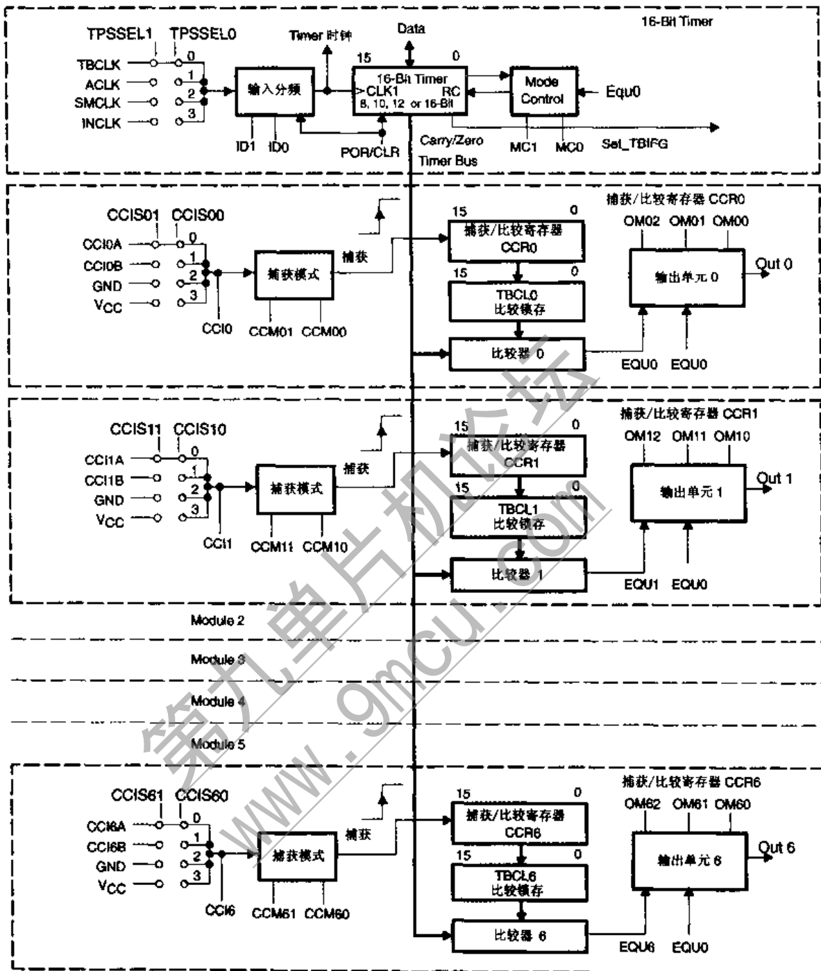
图 11.1 Timer_B 结构
