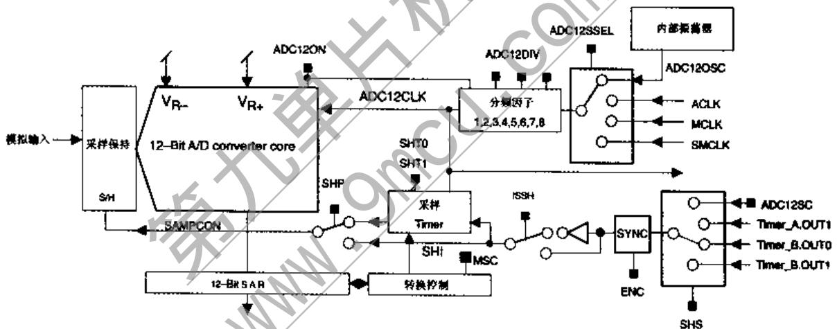
图 15.18 脉冲采样模式结构
