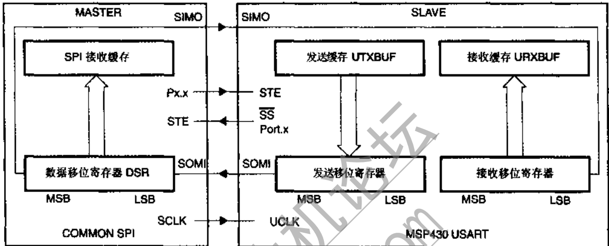
图 13.5 MSP430 的 USART 作为 3 线或 4 线连接的从机
