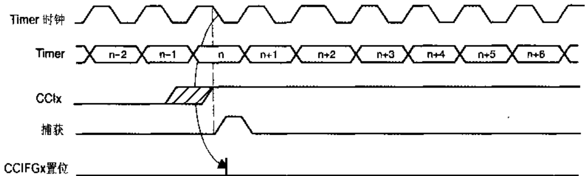
图 10.19 捕获信号
