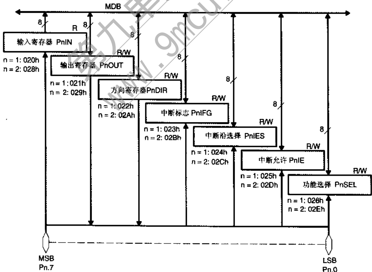
图 8.1 P1、P2 结构
