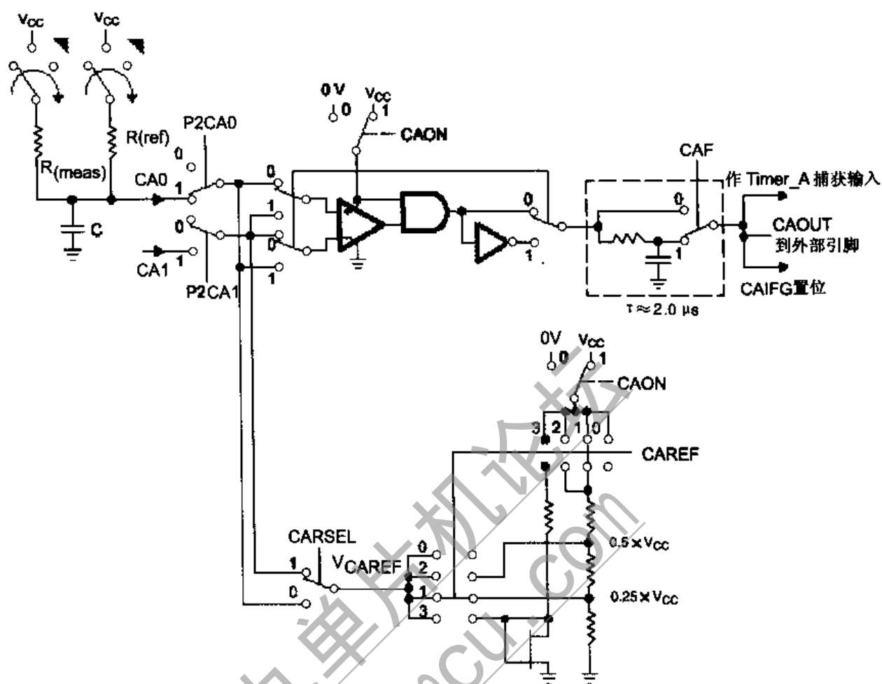
图 14.7 温度测量系统
