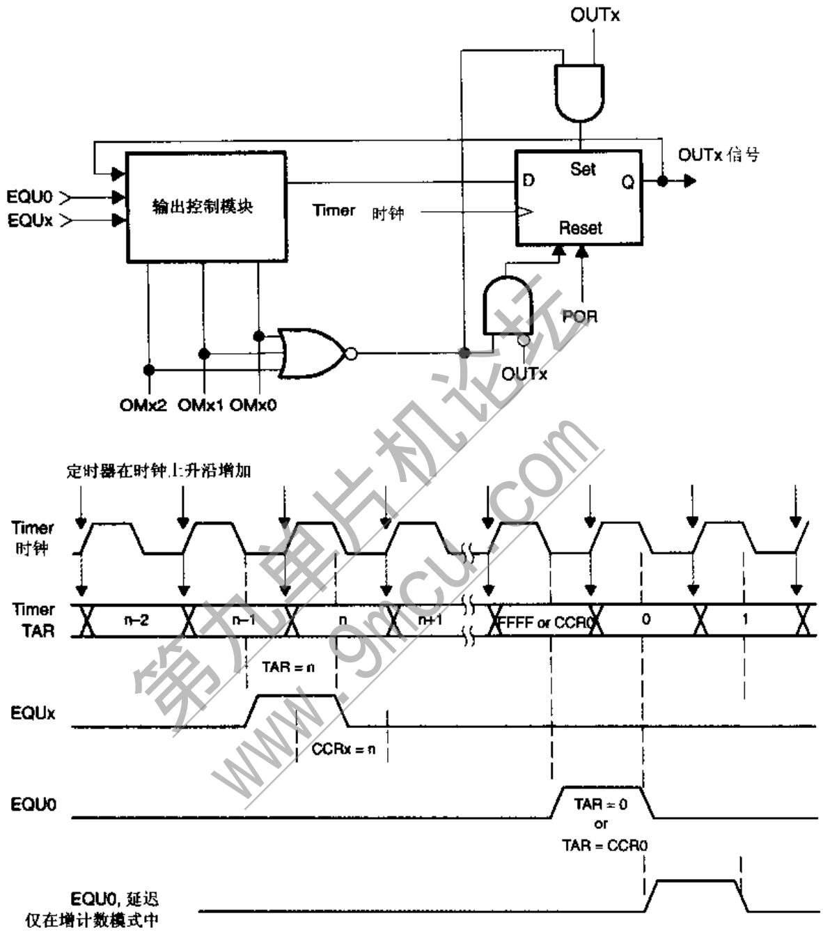
图 10.23 输出控制模块及时序
