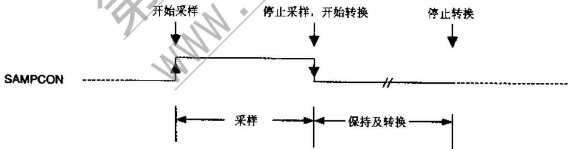
图 15.15 采样及转换时序
