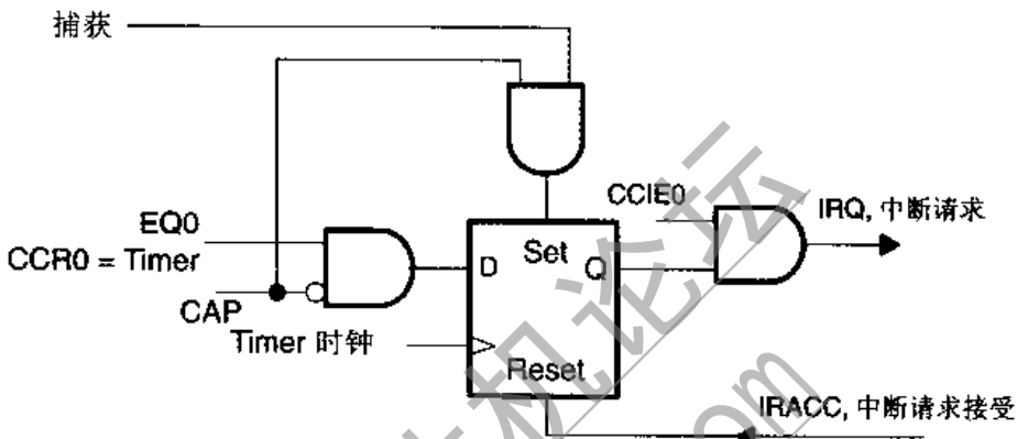
图 10.27 CCR0 中断标志
