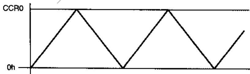
图 10.12 增/减计数模式
