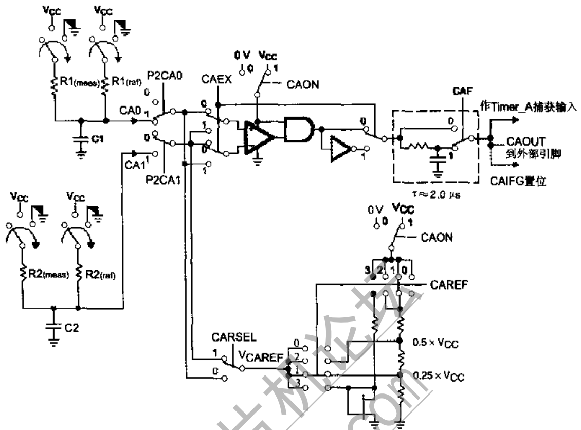
图 14.10 上通道经过 R1(\text{meas}) 测量温度
