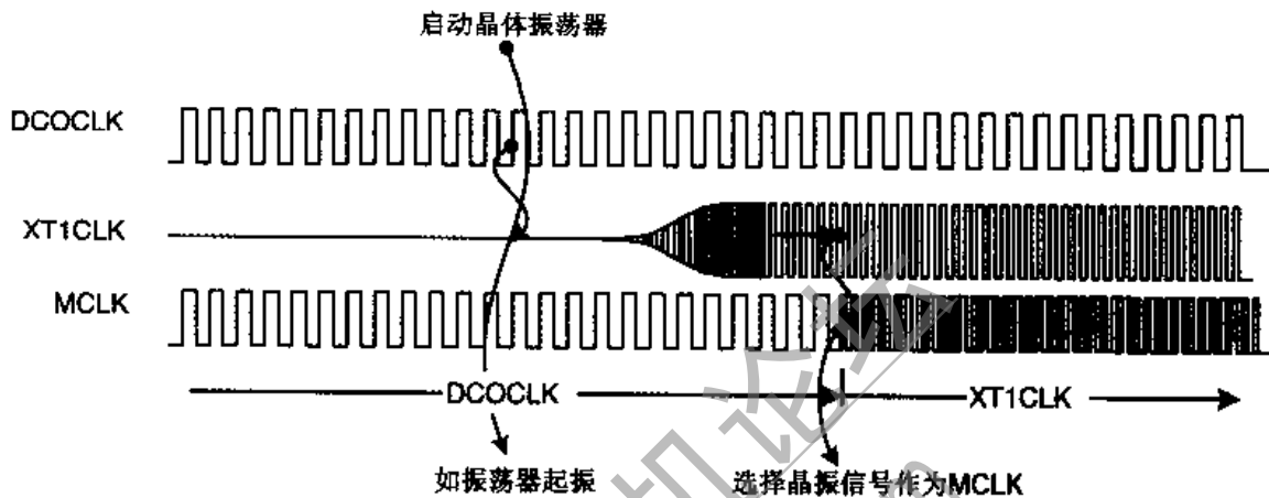
图 7.14 高频模式 LFXT1 用作 MCLK
