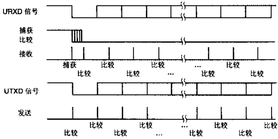
图 10.30 Timer_A 实现 UART 的时序
