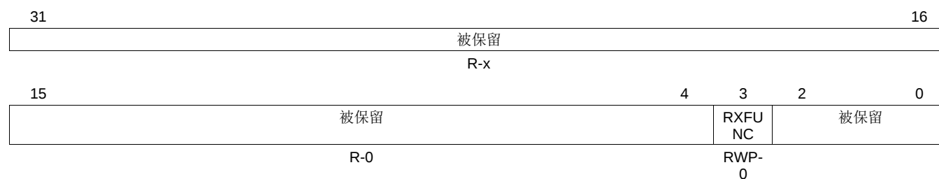
图 28. RX I/O 控制寄存器 (CANRIOC)
