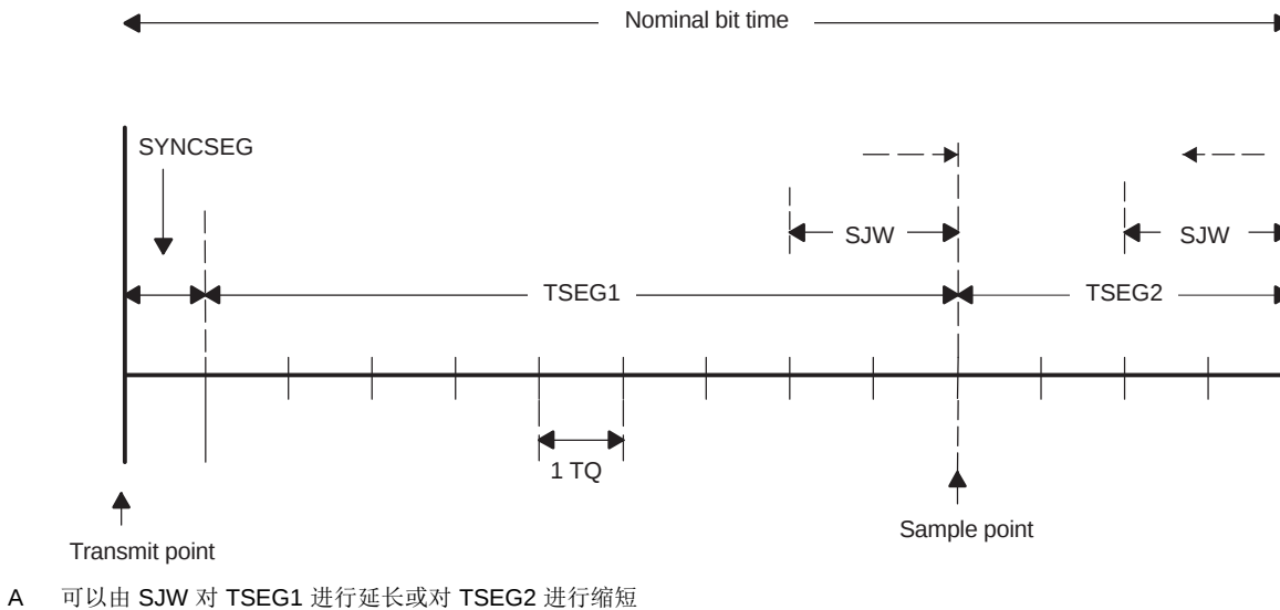
图 42. CAN 位时序
