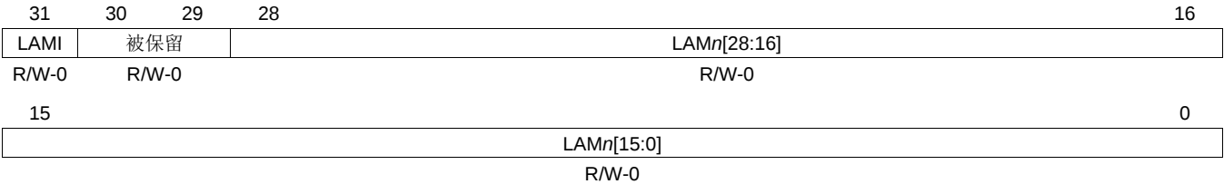
图 40. 本地接受屏蔽寄存器 (LAMn)
