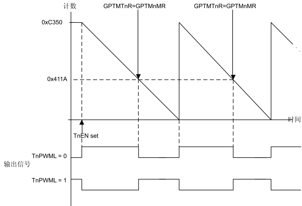
图 9-4. 16-位PWM模式实例
