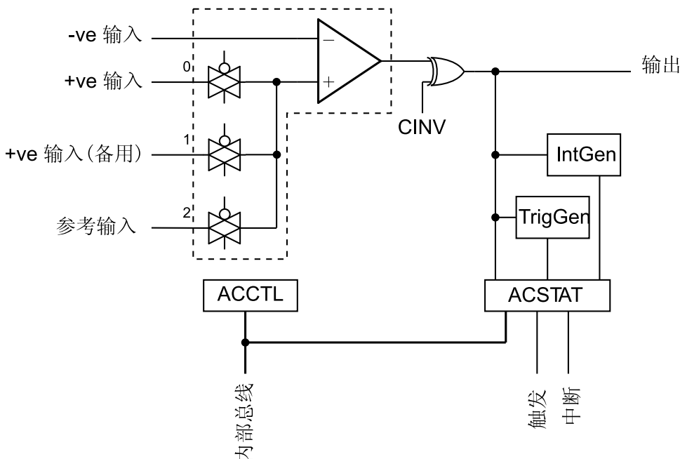
图 15-2. 比较单元的结构
