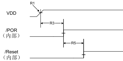
图 19-10. 上电复位时序
