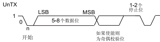
图 12-2. UART字符帧
