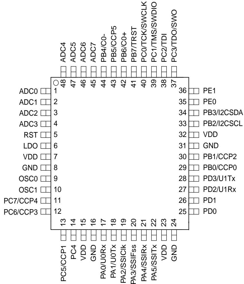
图 16-1. 管脚连接图
