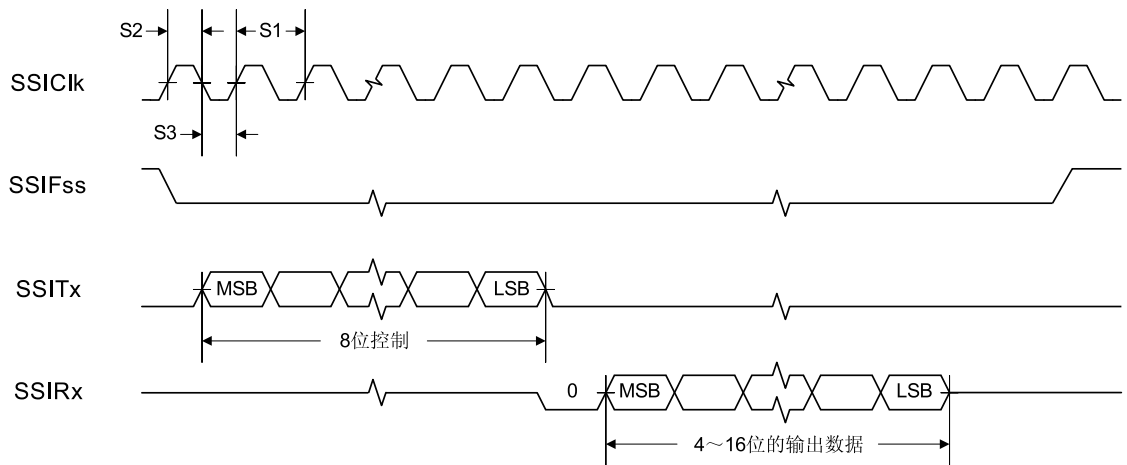
图 19-4. MICROWIRE 帧格式 (FRF=10) 的 SSI 时序, 单次传输
