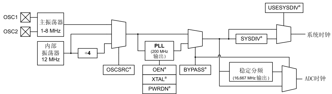
图 6-2. 主时钟树
