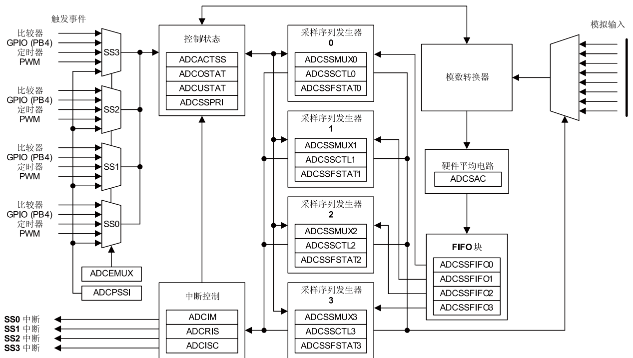
图 11-1. ADC模块框图
