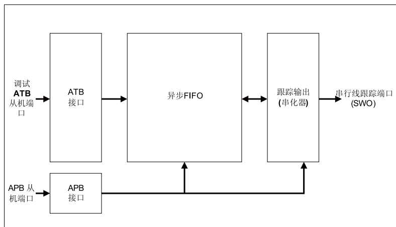
图 2-2. TPIU方框图
