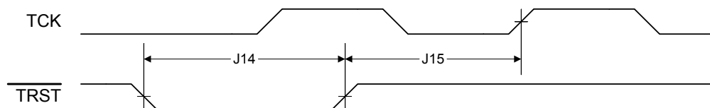
图 19-8. JTAG TRST 时序
