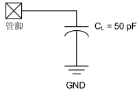
图 19-1. 负载条件
