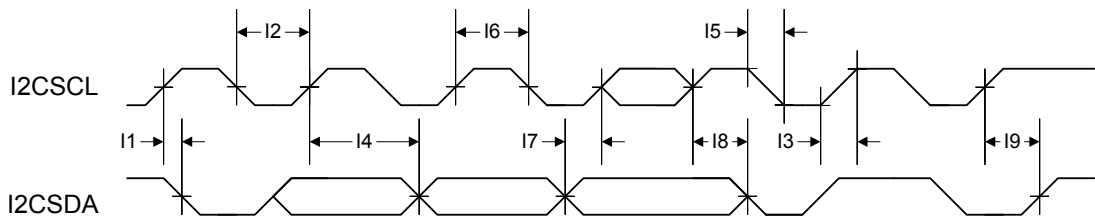
图 19-2. I 2 C时序
