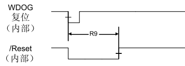
图 19-13. 看门狗复位时序
