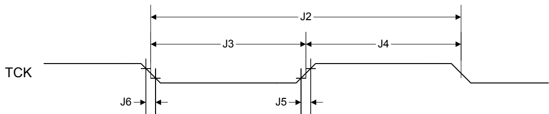
图 19-6. JTAG测试时钟输入时序
