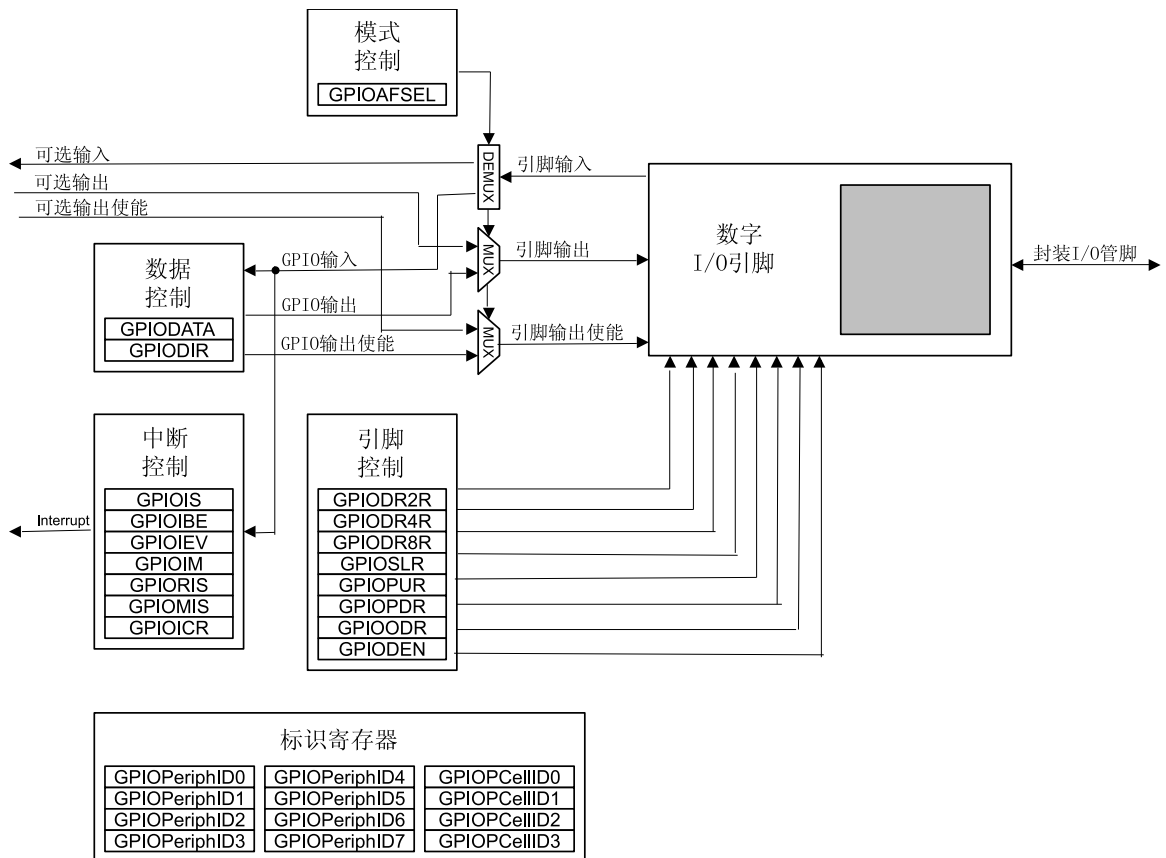
图 8-1. GPIO端口方框图
