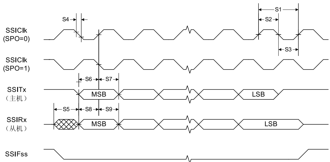
图 19-5. SPI 帧格式 (FRF=00), SPH=1
