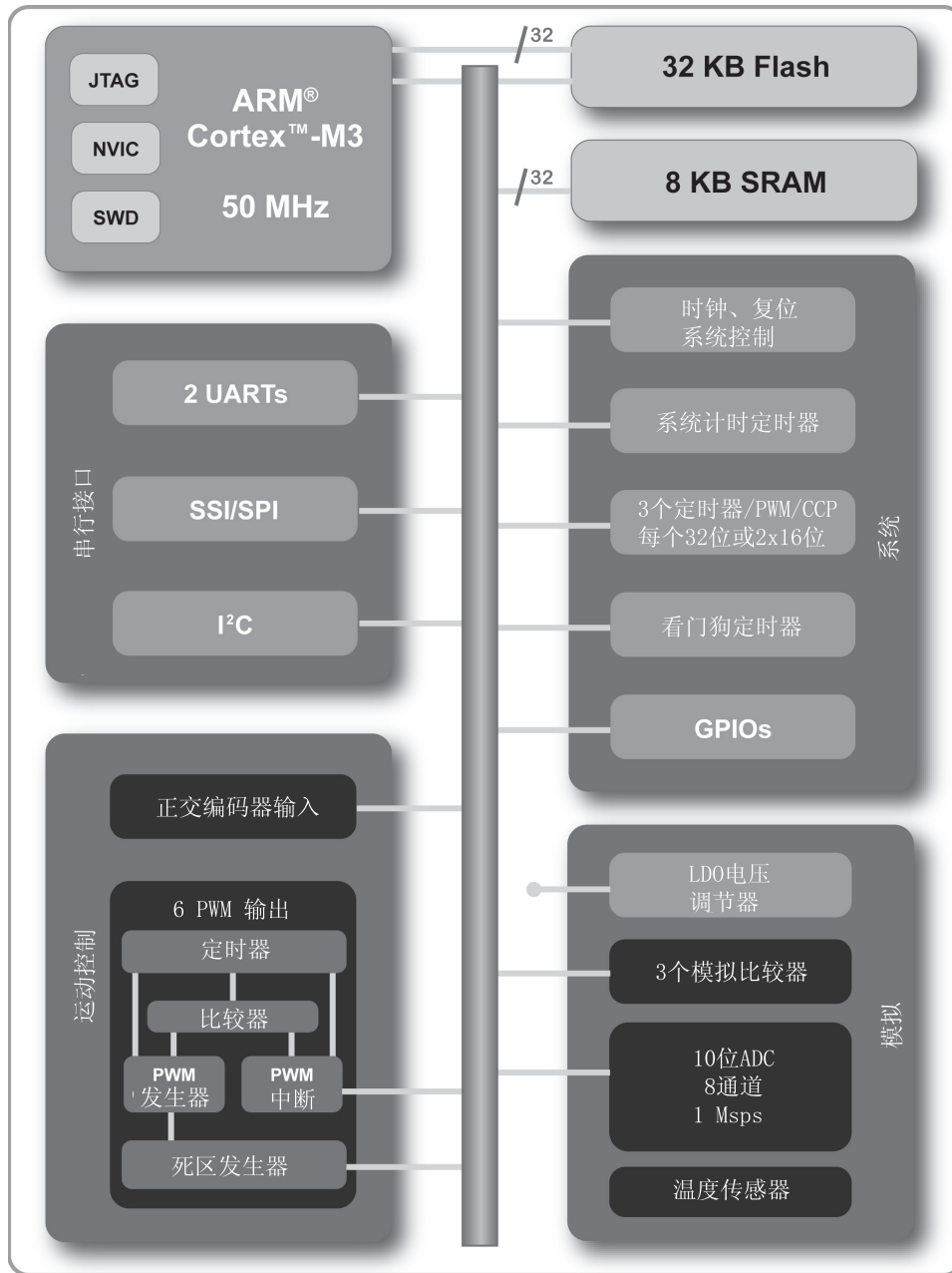
图 1-1. Stellaris® 600 系列高级方框图
