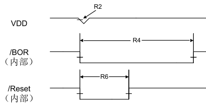
图 19-11. 掉电复位时序
