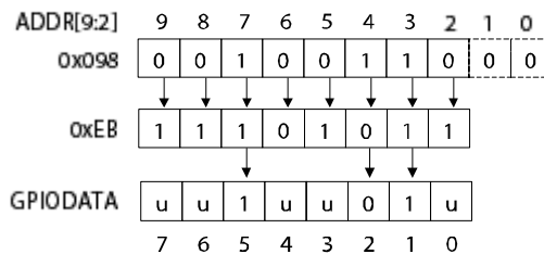
图 8.3 “GPIODATA 写”实例
