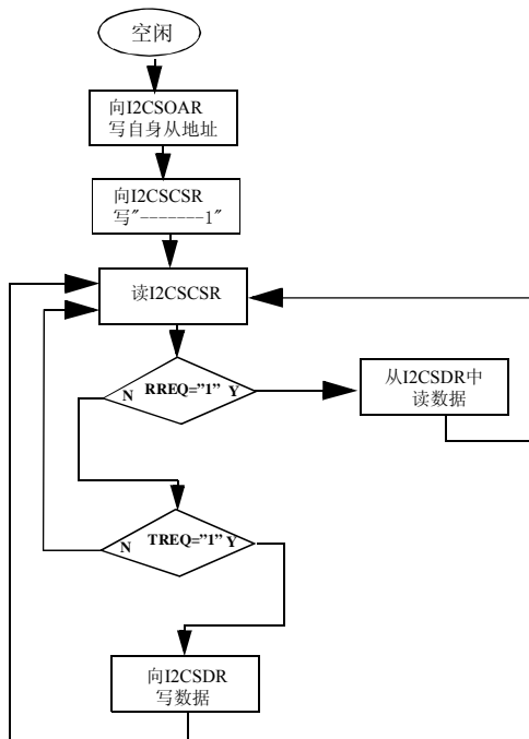
图 14.13 从机命令序列
