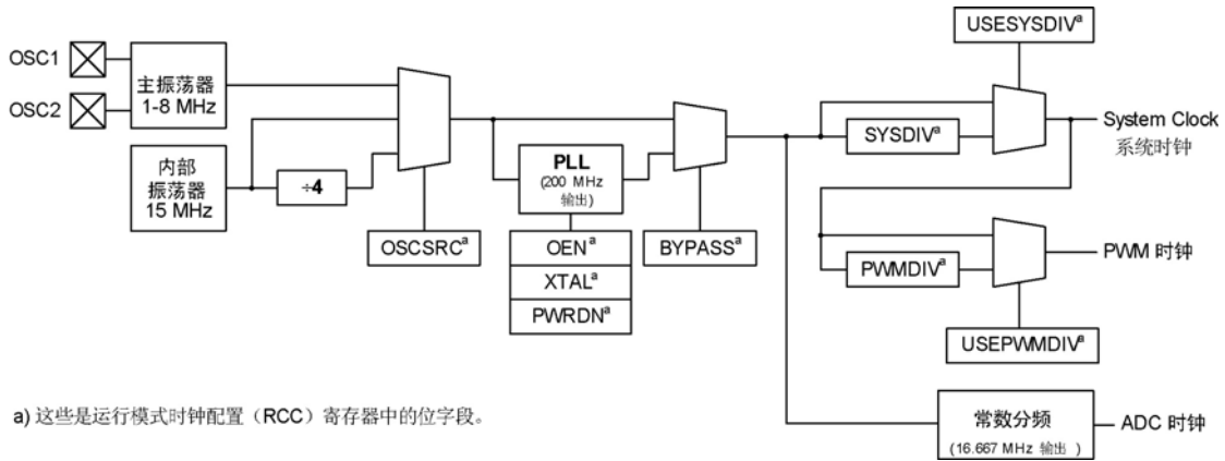
图 6.2 主时钟树
