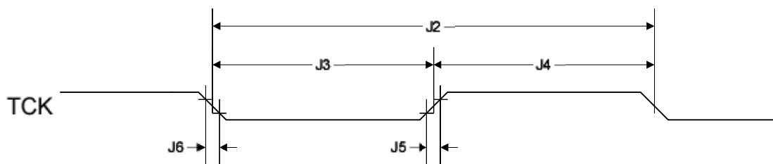
图 20.6 JTAG 测试时钟的输入时序
