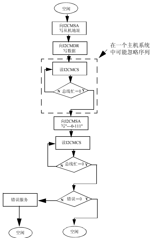
图 14.7 主机单次发送
