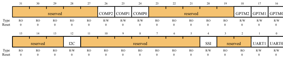
软件复位控制1 (SRCR1) Offset 0x044
