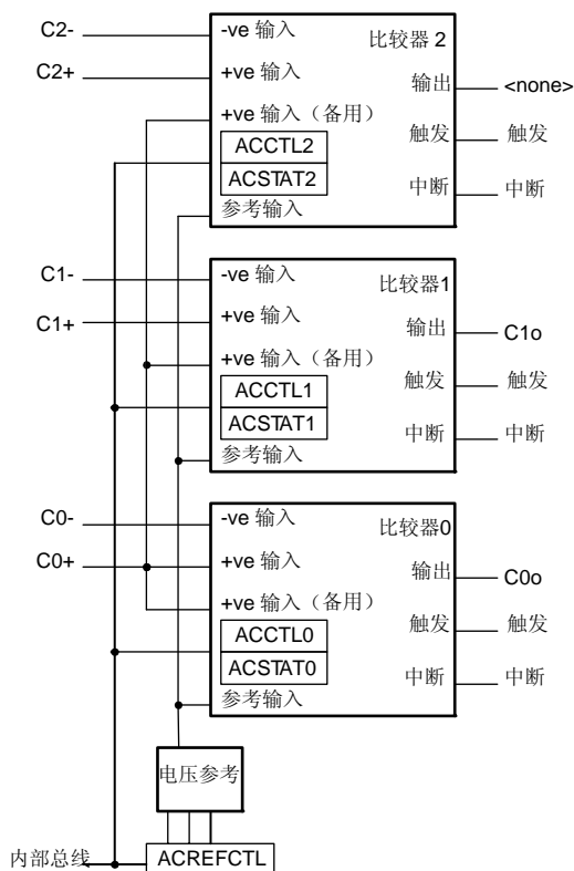
图 15.1 模拟比较器模块方框图
