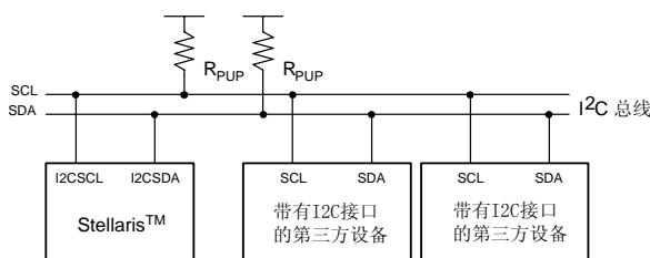
图 14.2 I 2 C 总线配置
