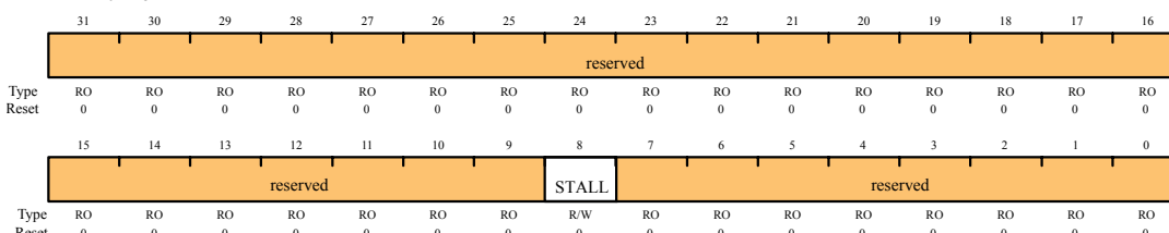
看门狗测试 (WDTTEST) 偏移量 0x418
