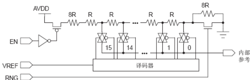
图 15.3 比较器内部参考的结构
