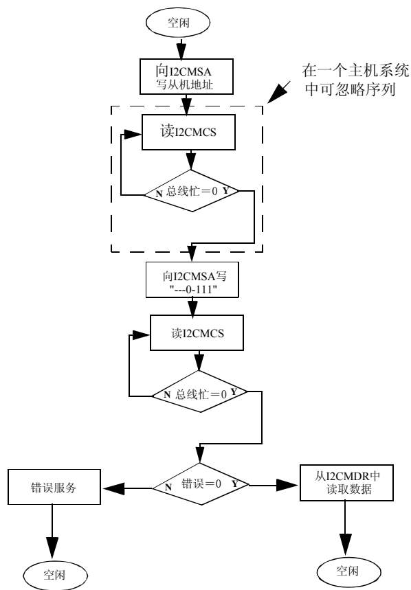
图 14.8 主机单次接收
