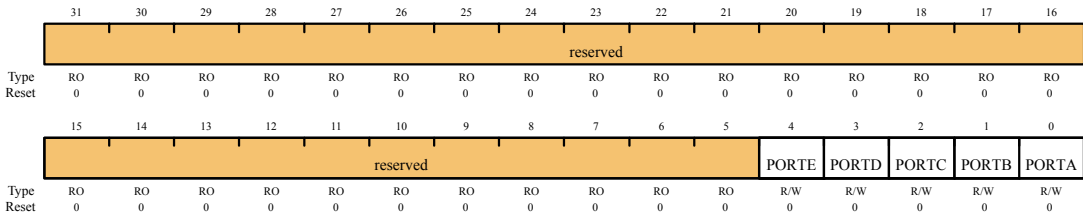
运行模式、睡眠模式和深度睡眠模式时钟门控 (RCGC2, SCGC2和 DCGC2) Offset 0x108, 0x118, and 0x128
