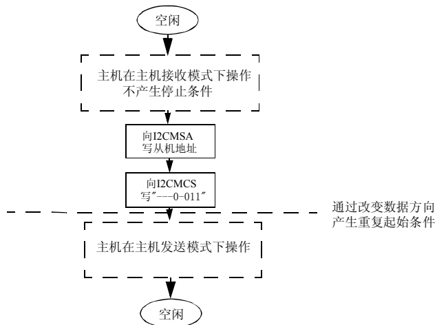
图 14.12 在突发接收后主机突发发送
