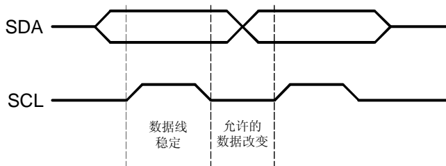
图 14.3 在 I 2 C 总线的位传输过程中的数据有效性
