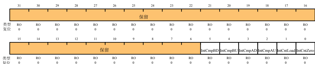
PWMn 原始中断状态 (PWMnRIS)
