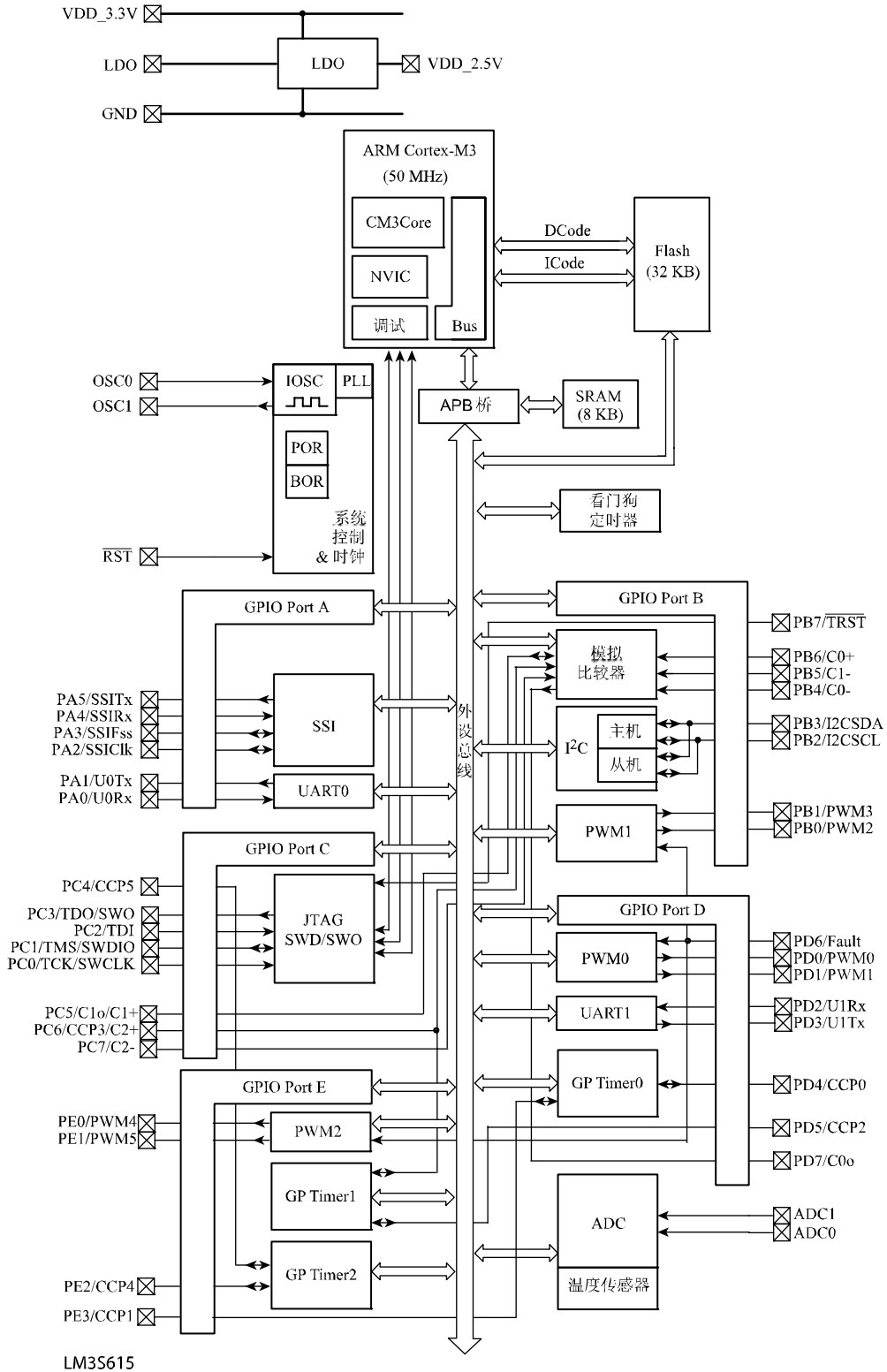
图 1.2 LM3S615 控制器系统级方框图
