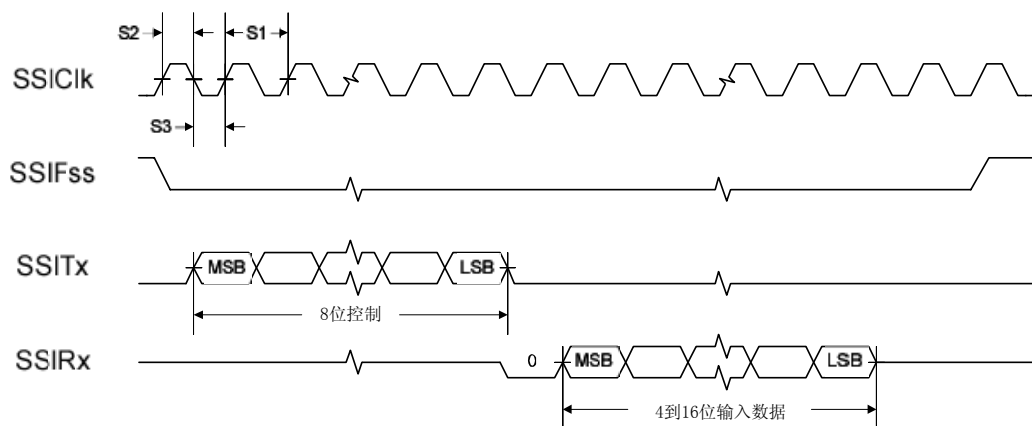
图 20.4 MICROWIRE 帧格式的 SSI 时序 (FRF=10), 单次传输
