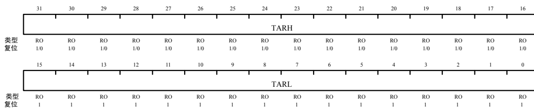
GPTM TimerA (GPTMTAR) 偏移量 0x048
