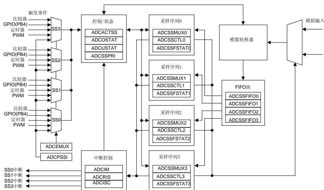
图 11.1 ADC 模块流程图
