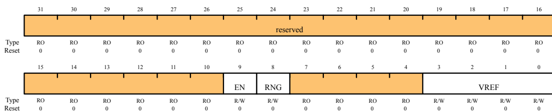
模拟比较器参考电压控制 (ACREFCTL) 偏移量 0x10
