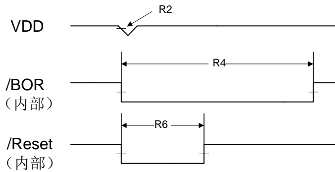
图 20.11 掉电 (brown-out) 复位时序
