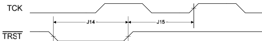
图 20.8 JTAG \overline{TRST} 时序
