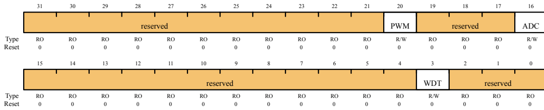
软件复位控制0 (SRCR0) 寄存器 偏移量 0x040
