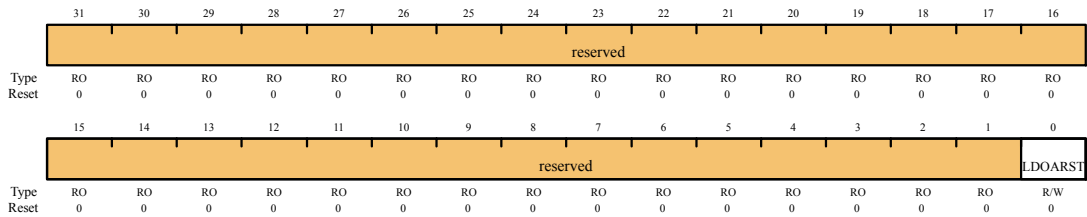
允许未调整LDO复位器件 (LDOARST) 寄存器 偏移量 0x160
