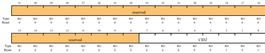
GPIO PrimeCell标识2 (GPIOCellID2) 寄存器 偏移量 0xFF8
