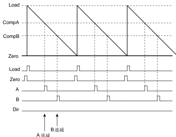
图 16.2 PWM 递减计数模式
