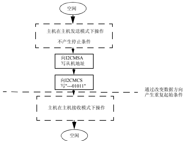
图 14.11 在突发发送后主机突发接收
