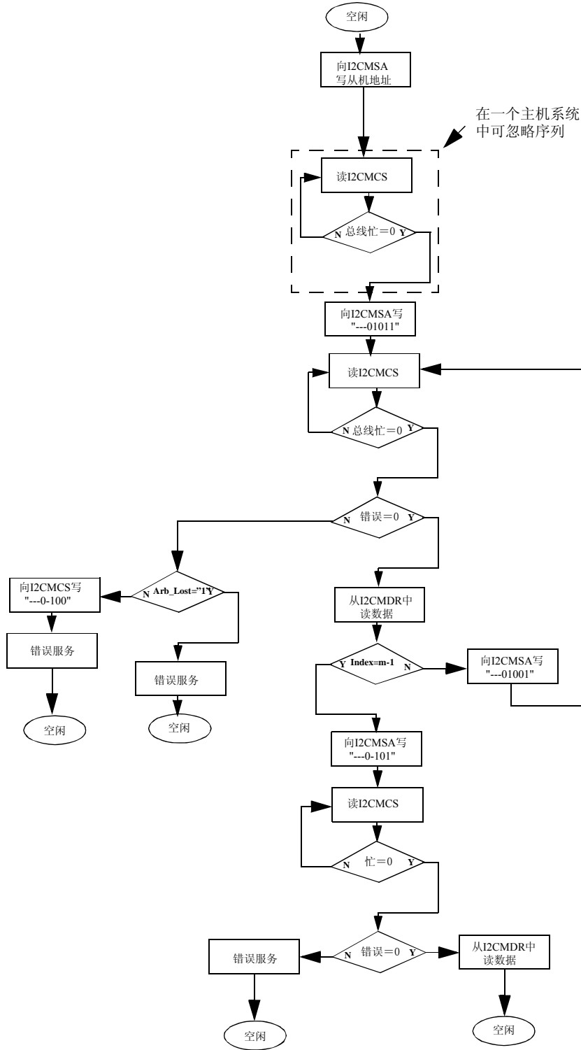
图 14.10 主机突发接收
