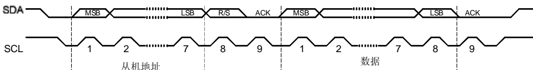
图 14.5 带 7 位地址的完整数据传输
