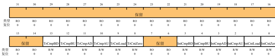
PWMn 中断/触发使能(PWMnINTEN)
