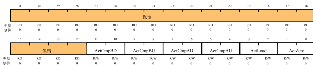
PWMn 发生器A控制 (PWMnGENA)
