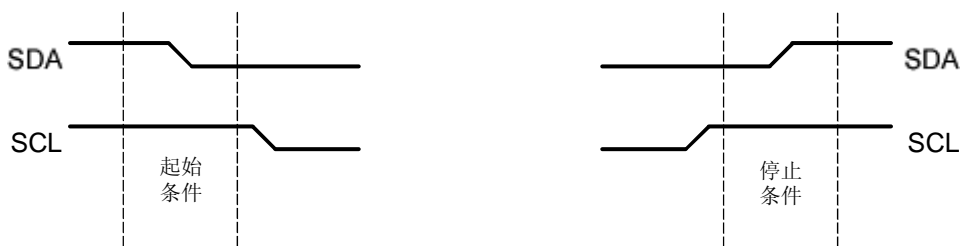
图 14.4 起始和停止条件
