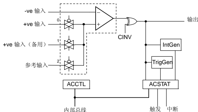
图 15.2 比较器单元的结构
