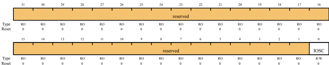
深度-睡眠时钟配置(DSLPCCLKCFG)寄存器 偏移量 0x144
