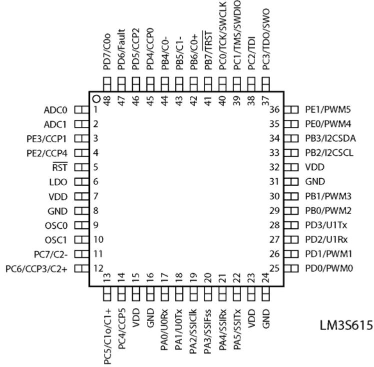
图 17.1 管脚连接图
