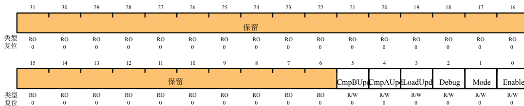
PWMn 控制 (PWMnCTL)
