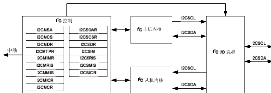
图 14.1 I 2 C 框图
