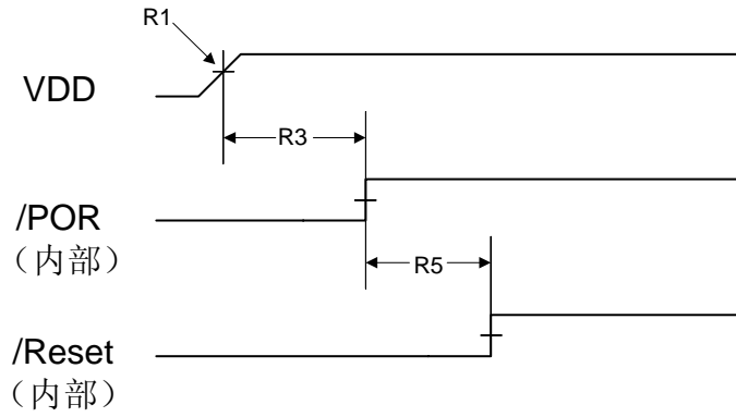
图 20.10 上电复位时序
