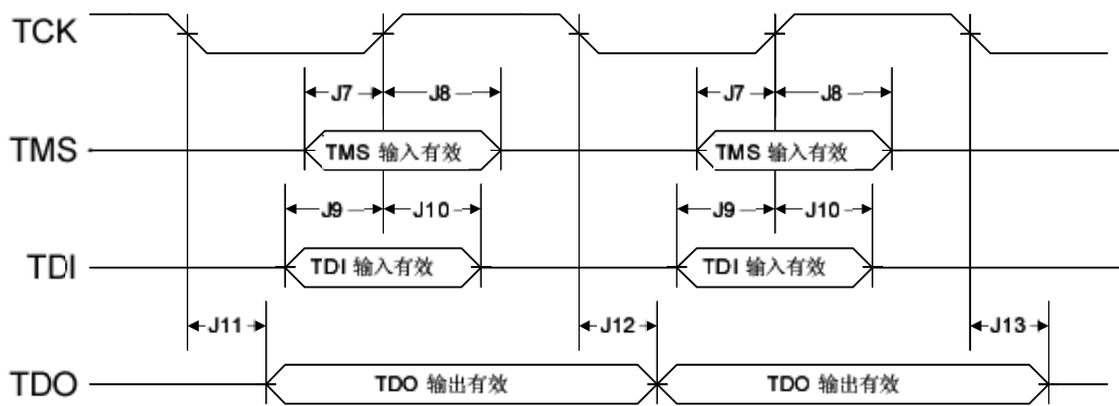
图 20.7 JTAG 测试访问端口 (TAP) 的时序
