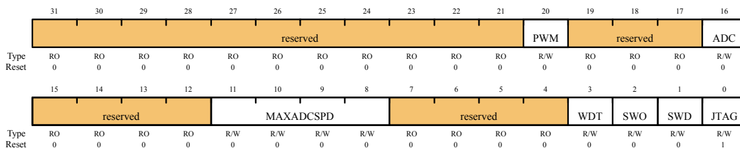
运行-模式、睡眠-模式和深度-睡眠-模式时钟门控0 (RCGC0、SCGC0和DCGC0) 寄存器 偏移量 0x100、0x110、0x120
