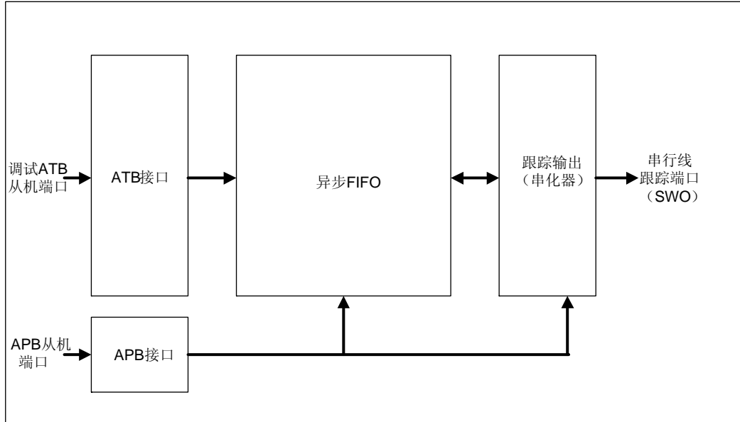
图 2.2 TPIU 方框图
