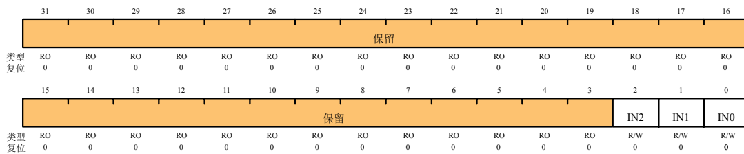
模拟比较器中断使能 (ACINTEN) 偏移量 0x08
