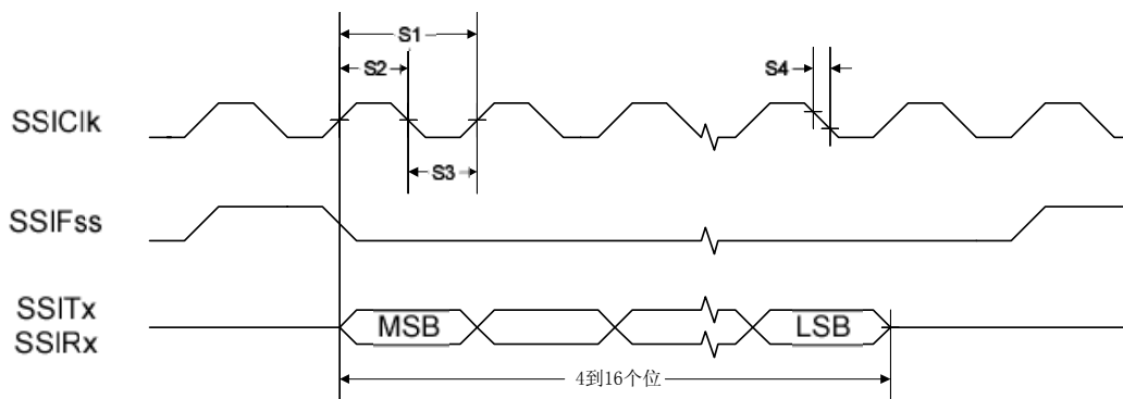
图 20.3 TI 帧格式 (FRF=01) 的 SSI 时序, 单次传输的时间测量
