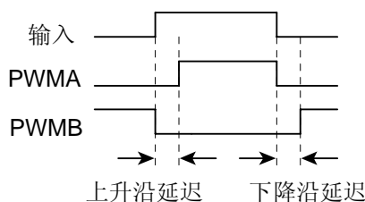
图 16.5 PWM 死区发生器
