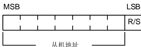
图 14.6 首字节的 R/S 位
