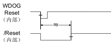
图 20-15. 看门狗复位时序
