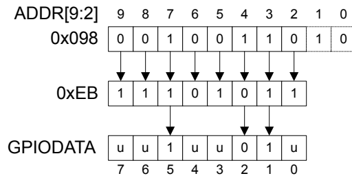
图 9-2. GPIODATA 写实例
