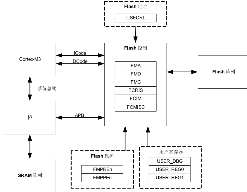
图 8-1. Flash方框图
