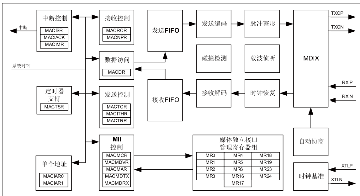
图 15-1. 以太网控制器方框图
