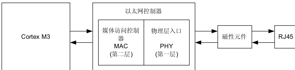
图 15-2. 以太网控制器
