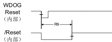
图 22-14. 看门狗复位时序
