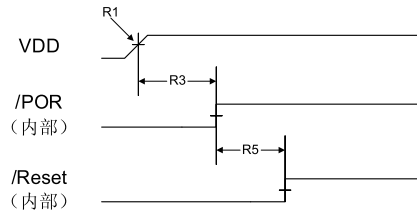
图 22-12. 掉电复位时序
