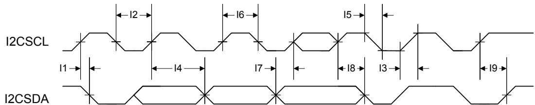
图 22-2. I 2 C时序
