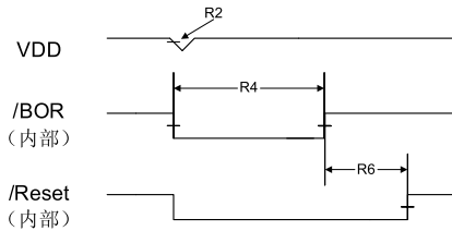
图 22-13. 软件复位时序
