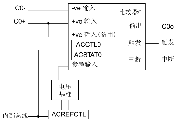
图 17-1. 模拟比较器模块的结构图
