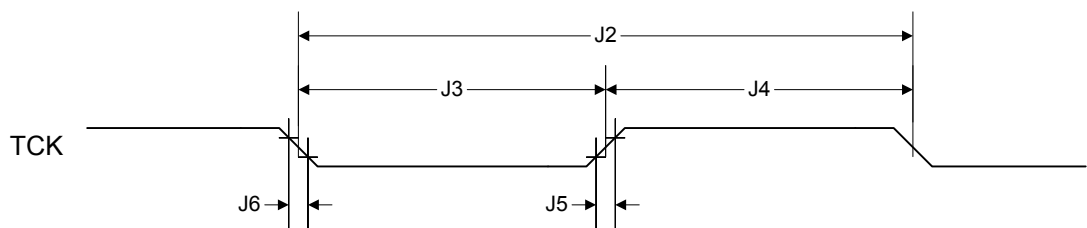
图 22-7. JTAG测试时钟输入时序
