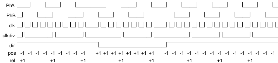
图 19-2. 正交编码器和速度预分频器的操作
