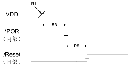
图 23-13. 掉电复位时序
