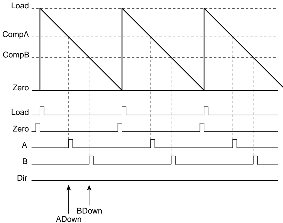
图 18-2. PWM递减计数模式
