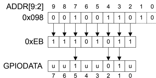
图 9-1. GPIODATA 写实例
