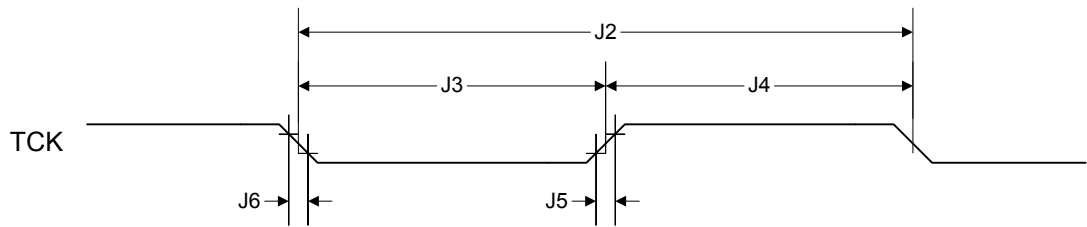
图 23-8. JTAG测试时钟输入时序
