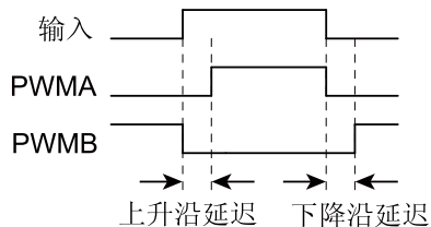
图 18-5. PWM死区发生器
