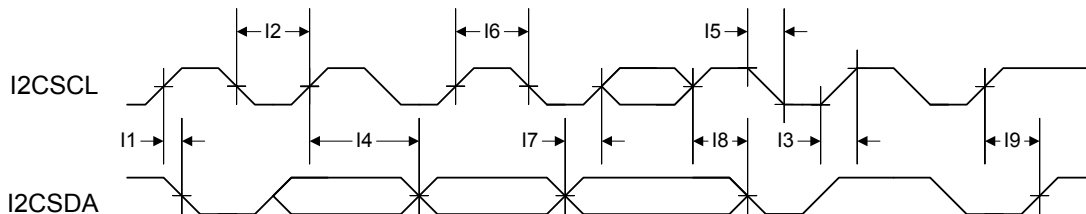
图 23-2. I 2 C时序
