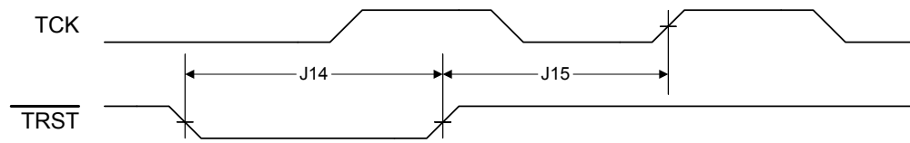
图 23-10. JTAG TRST时序
