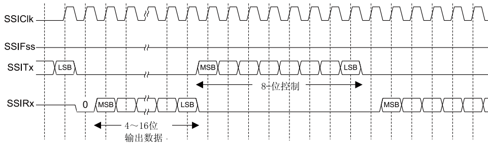
图 14-11. MICROWIRE的帧格式 (连续传输)
