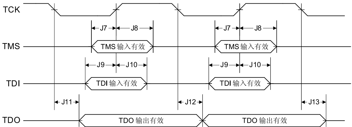
图 23-9. JTAG测试访问端口 (TAP) 时序
