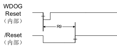
图 23-15. 看门狗复位时序
