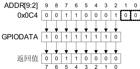
图 9-2. GPIODATA 读实例
