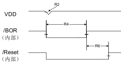
图 23-14. 软件复位时序
