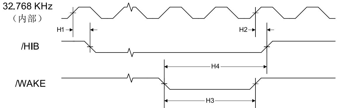
图 23-4. 休眠模块时序
