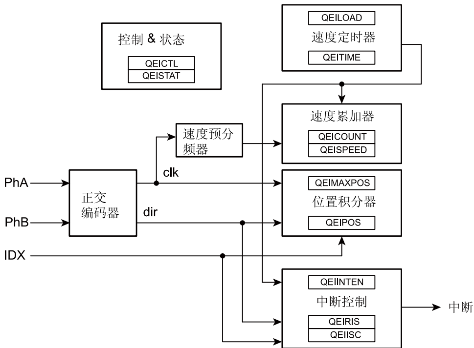
图 19-1. QEI结构图
