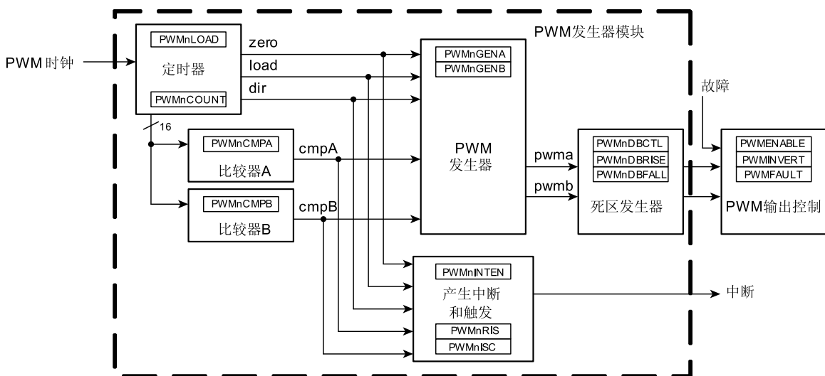
图 18-1. PWM 模块的结构图
