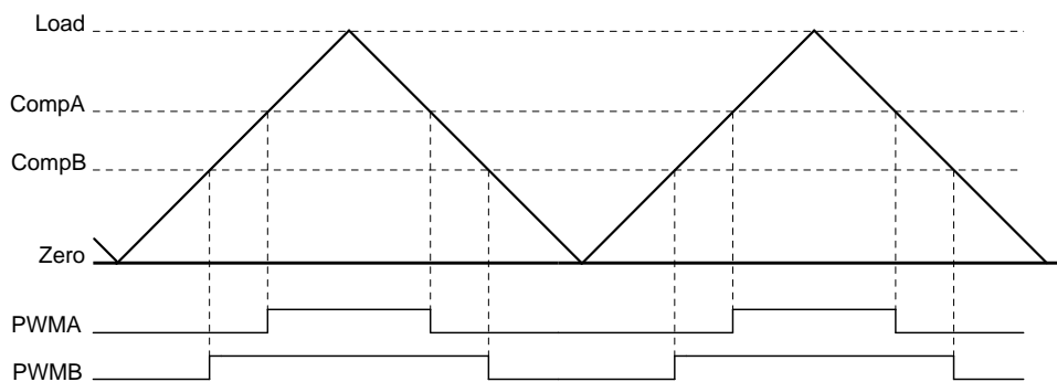
图 18-4. 在先递增后递减计数模式中产生PWM信号
