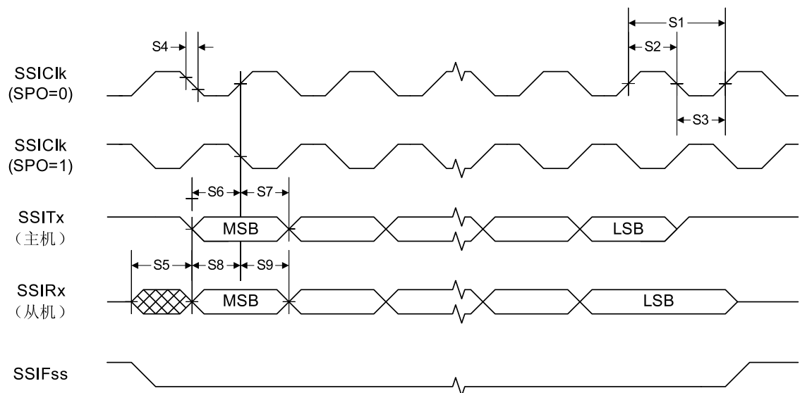
图 23-7. SPI 帧格式 (FRF=00), SPH=1
