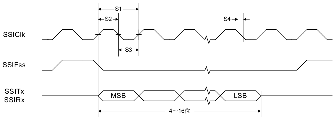
图 23-5. TI帧格式 (FRF=01) 的SSI时序, 单次传输的时序测量
