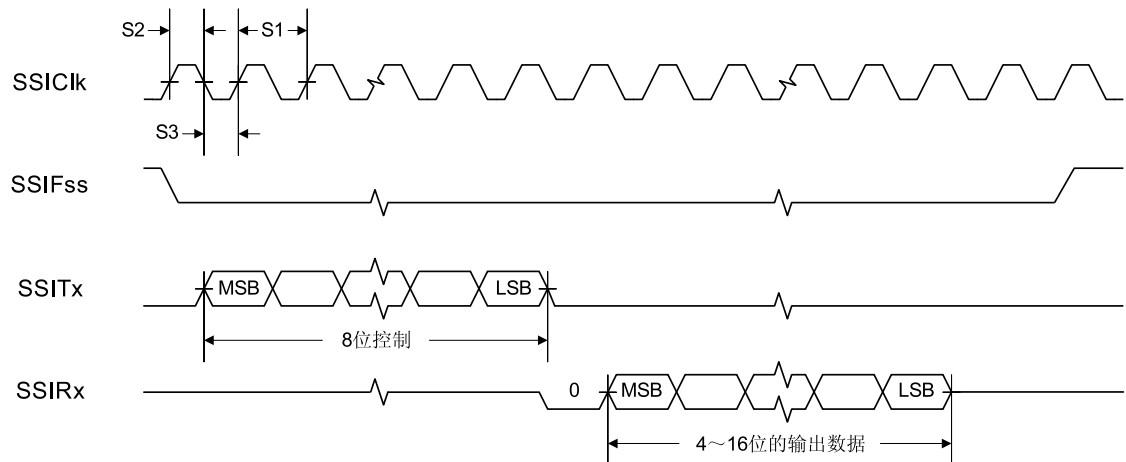
图 23-6. MICROWIRE 帧格式 (FRF=10) 的 SSI 时序, 单次传输
