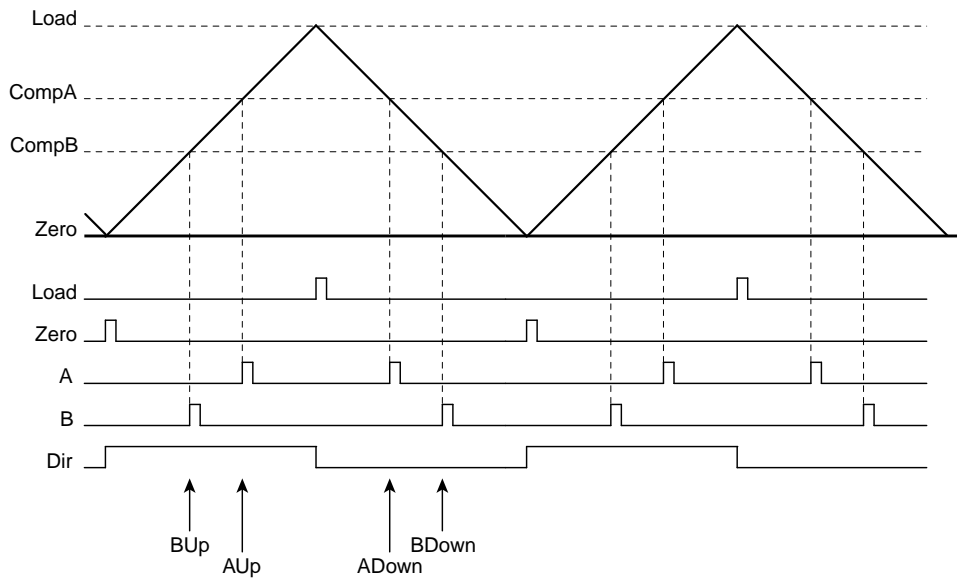
图 18-3. PWM先递增后递减计数模式
