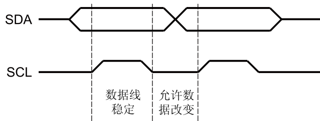
图 15-6. 在 I 2 C 总线的位传输过程中的数据有效性
