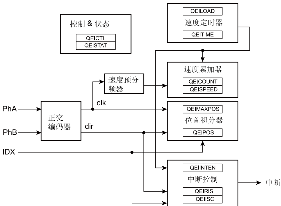
图 20-1. QEI结构图
