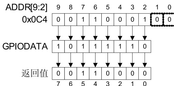
图 9-3. GPIODATA 读实例
