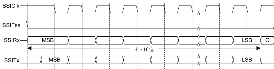
图 13-7. SPO=1和SPH=0时Freescale SPI的帧格式（单次传输）
