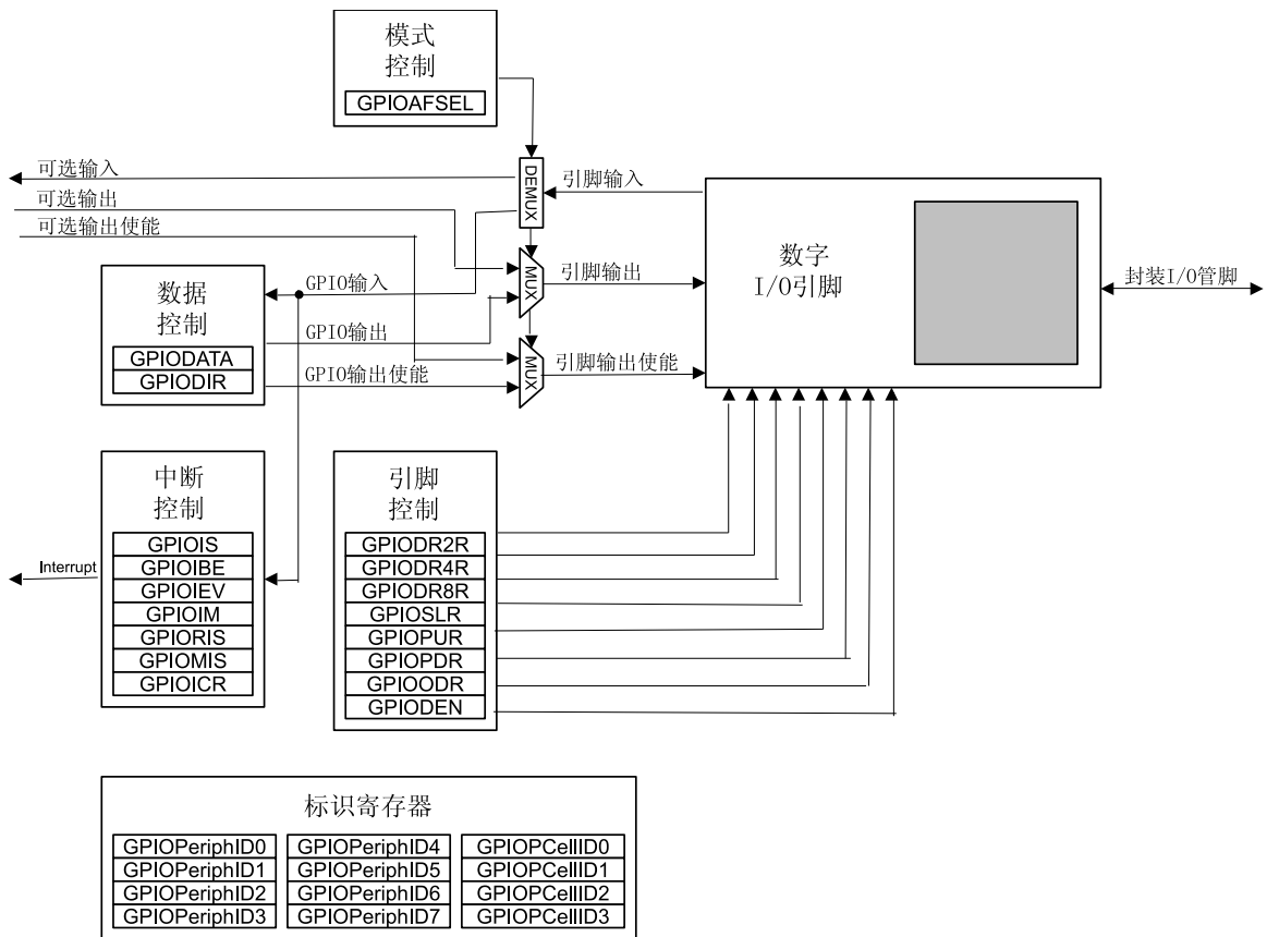
图 8-2. GPIO端口方框图
