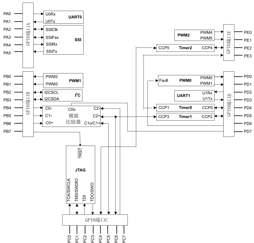
图 8-1. GPIO 模块框图
