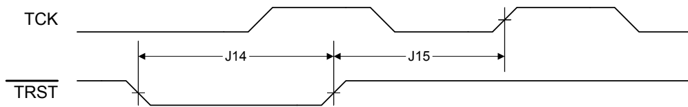
图 20-8. JTAG TRST 时序
