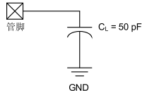
图 20-1. 负载条件
