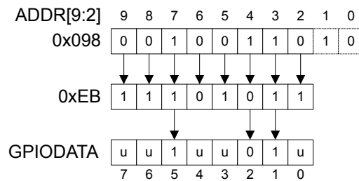
图 8-3. GPIODATA 写实例
