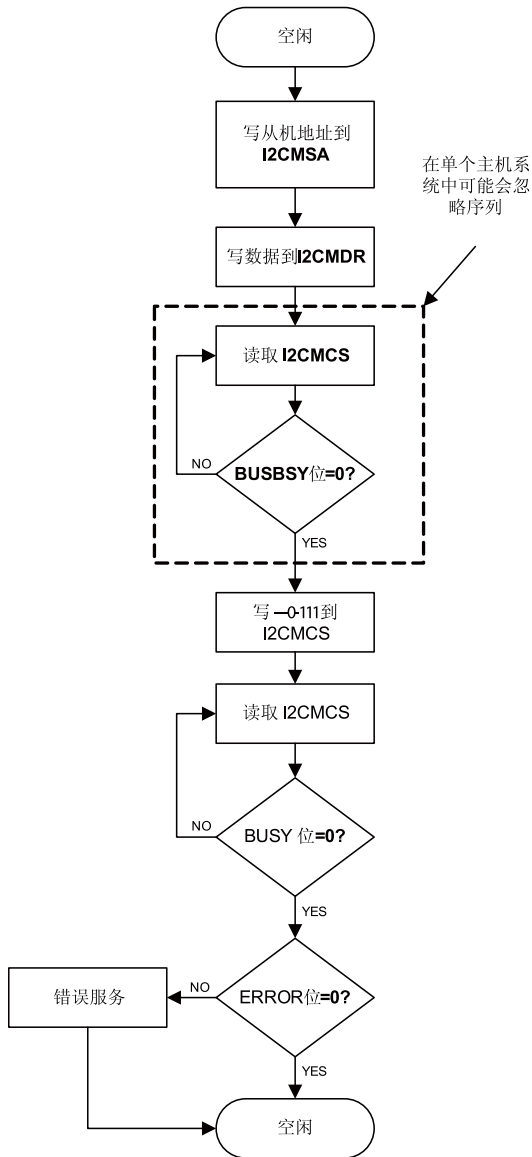
图 14-7. 主机单次发送
