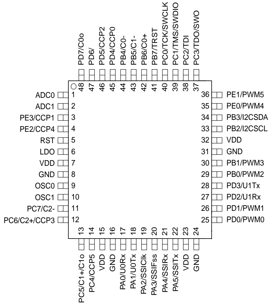
图 17-1. 管脚连接图
