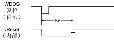
图 20-13. 看门狗复位时序
