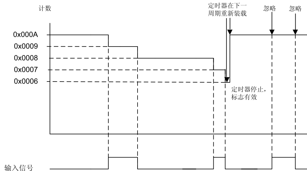
图 9-2. 16位输入边沿计数模式实例
