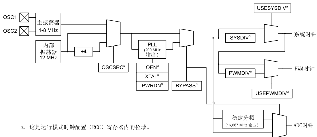
图 6-2. 主时钟树
