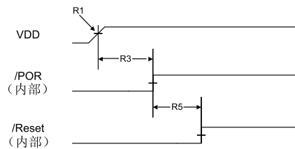
图 20-10. 上电复位时序
