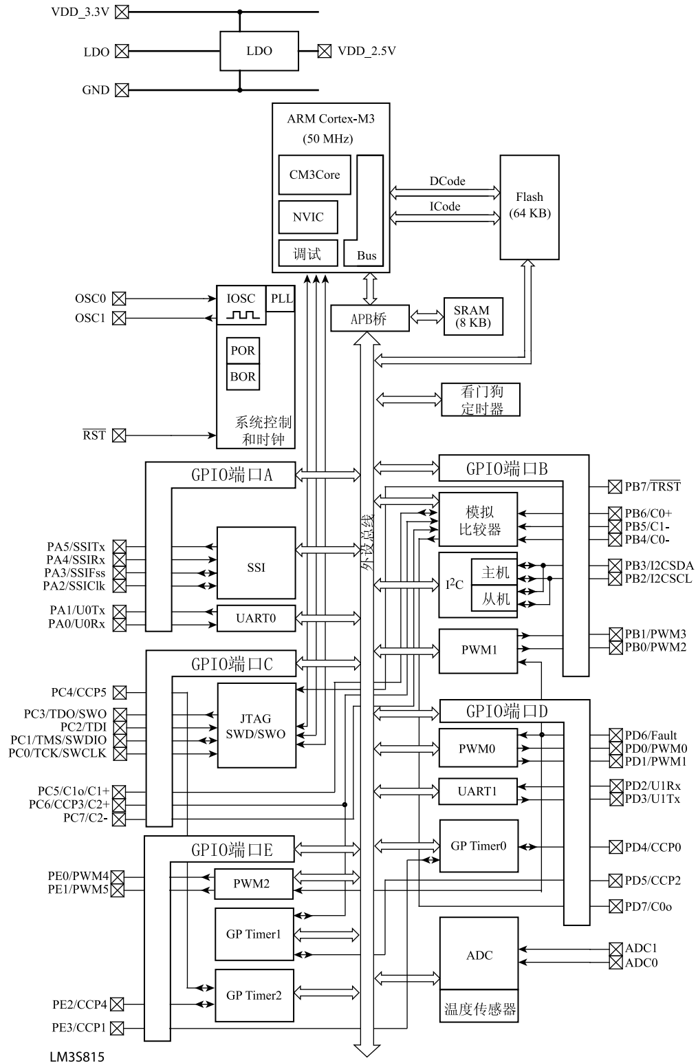
图 1-2. LM3S815 控制器系统级方框图
