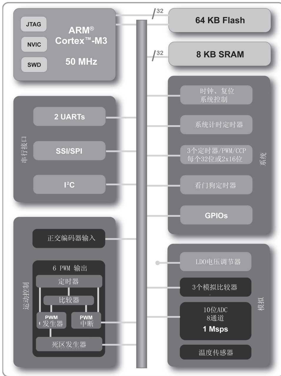
图 1-1. Stellaris® 800 系列高级方框图
