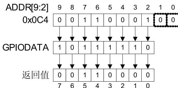
图 8-4. GPIODATA 读实例
