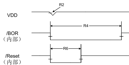
图 20-11. 掉电复位时序
