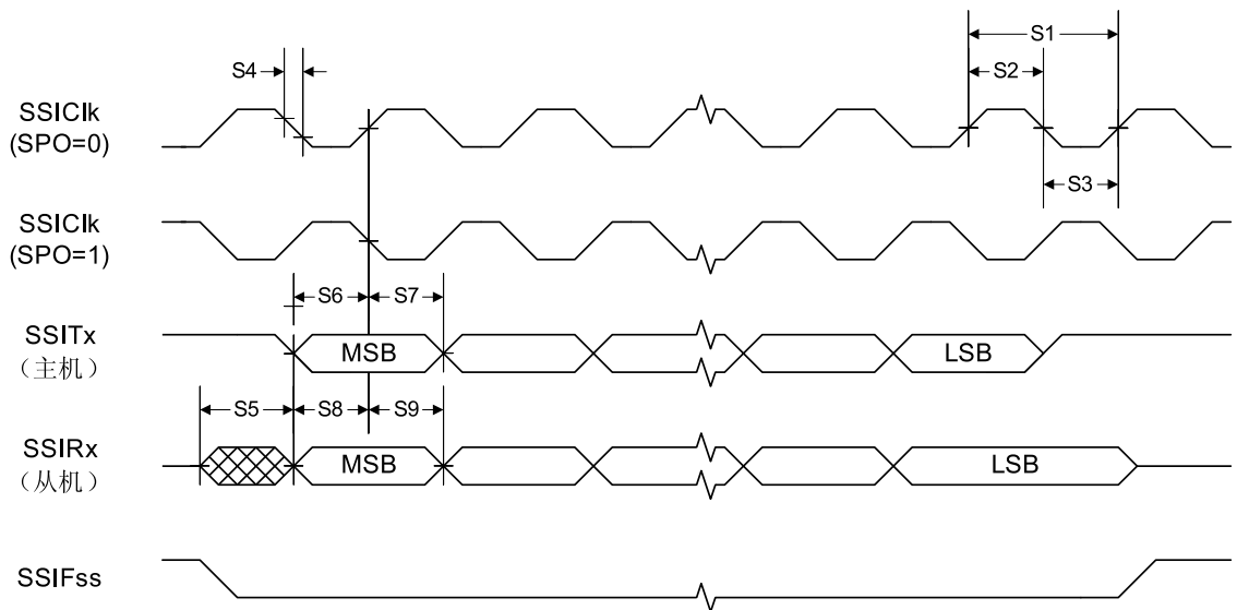
图 20-5. SPI帧格式 (FRF=00), SPH=1
