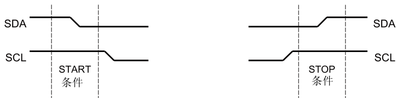
图 14-3. 起始和停止条件
