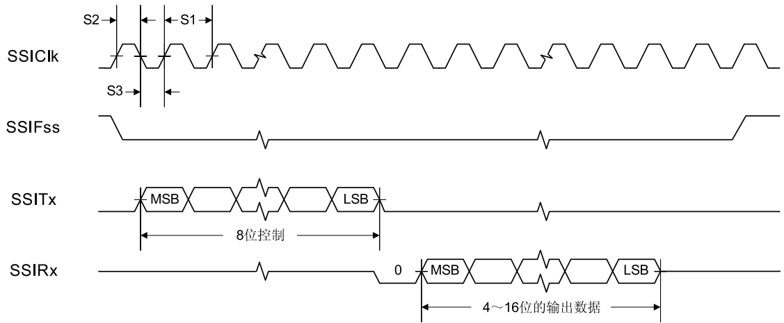
图 20-4. MICROWIRE帧格式 (FRF=10) 的SSI时序, 单次传输
