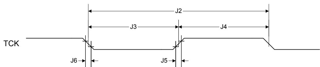
图 20-6. JTAG测试时钟输入时序
