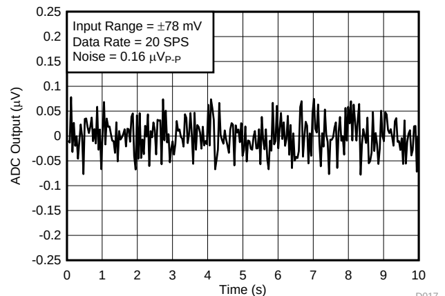
ADC 转换噪声
