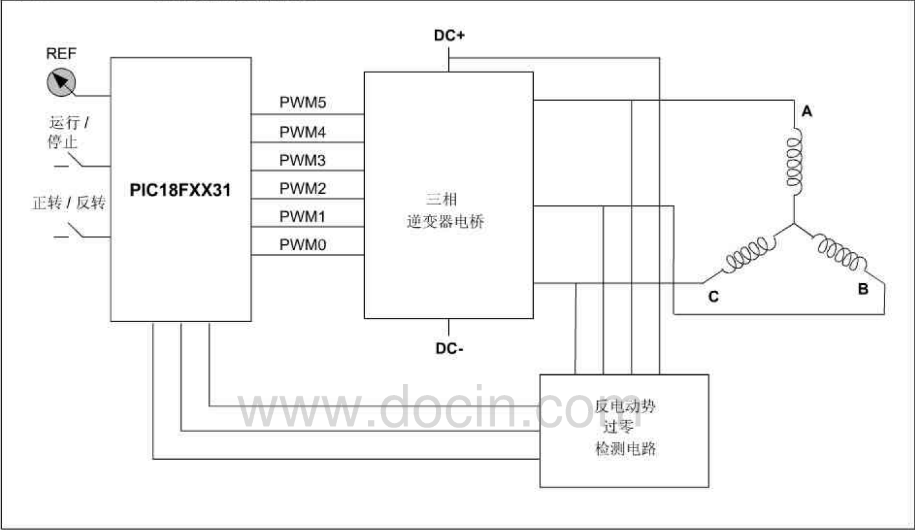
图 10: 无传感器控制框图
