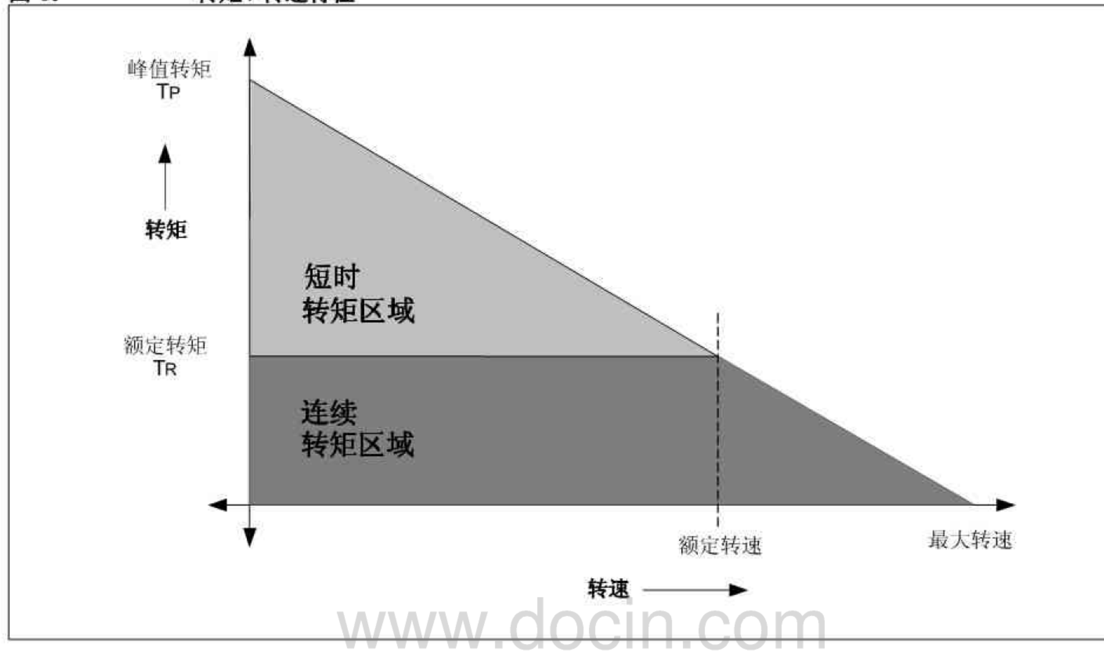
图 6: 转矩 / 转速特性
