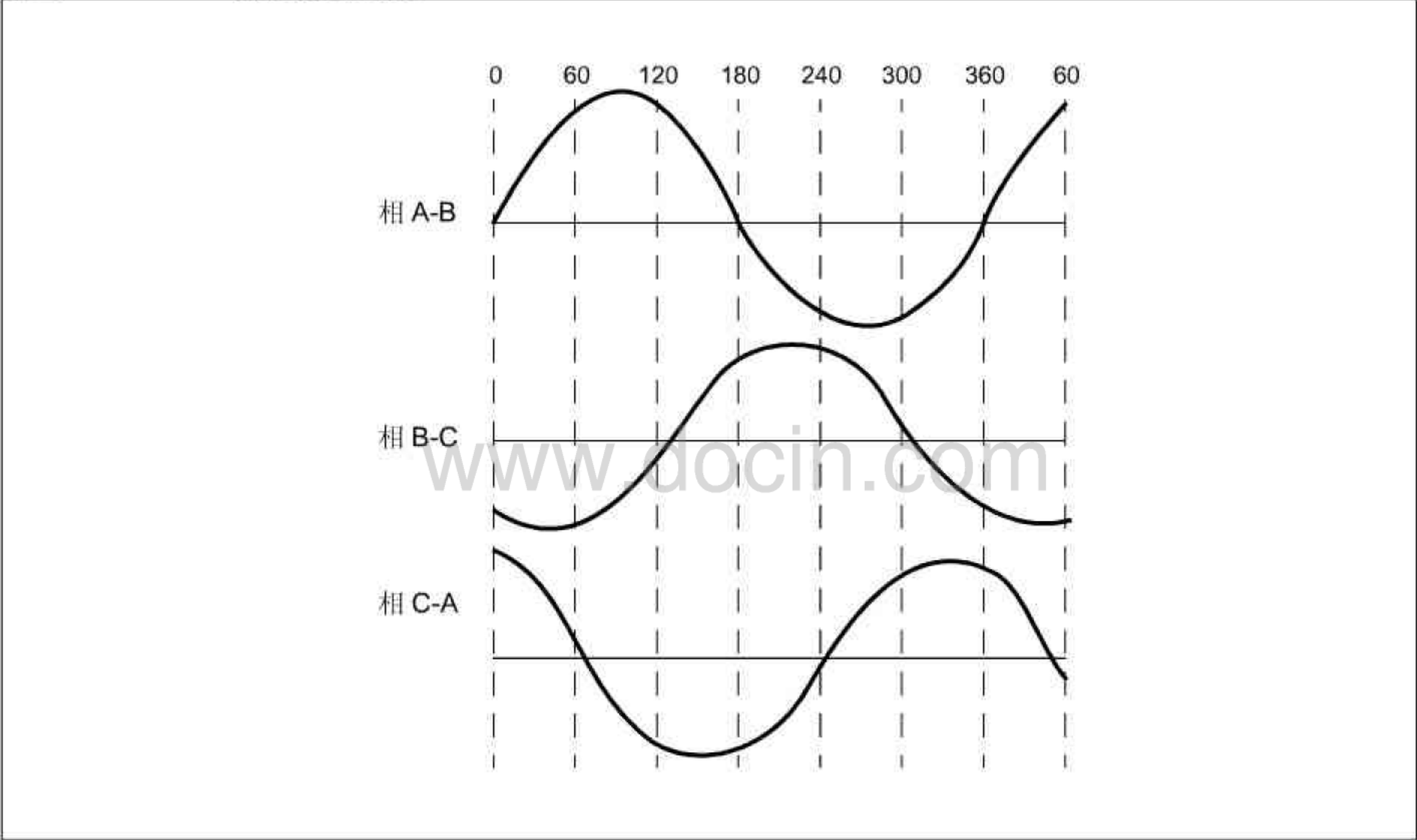
图 2: 正弦反电动势
