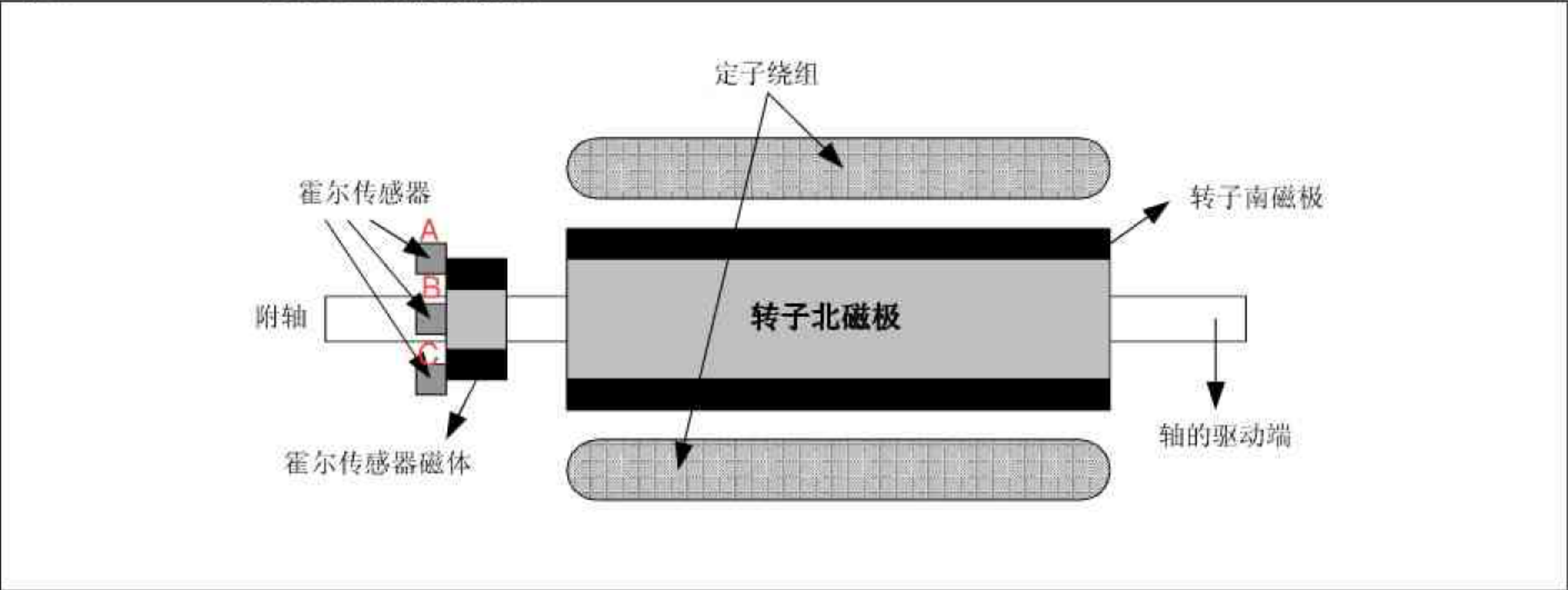
图 5: BLDC 电机横截面
