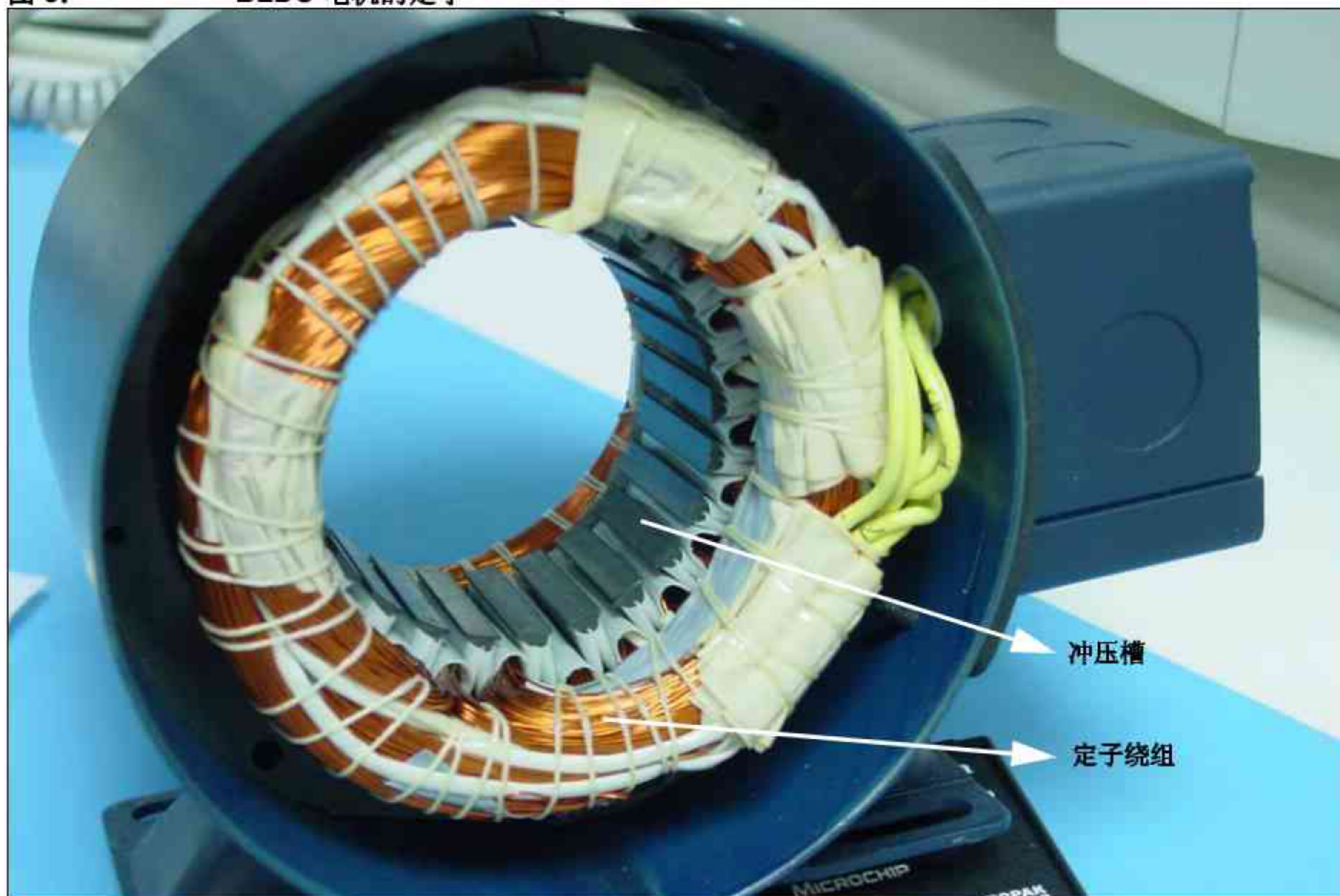
图 3: BLDC 电机的定子
