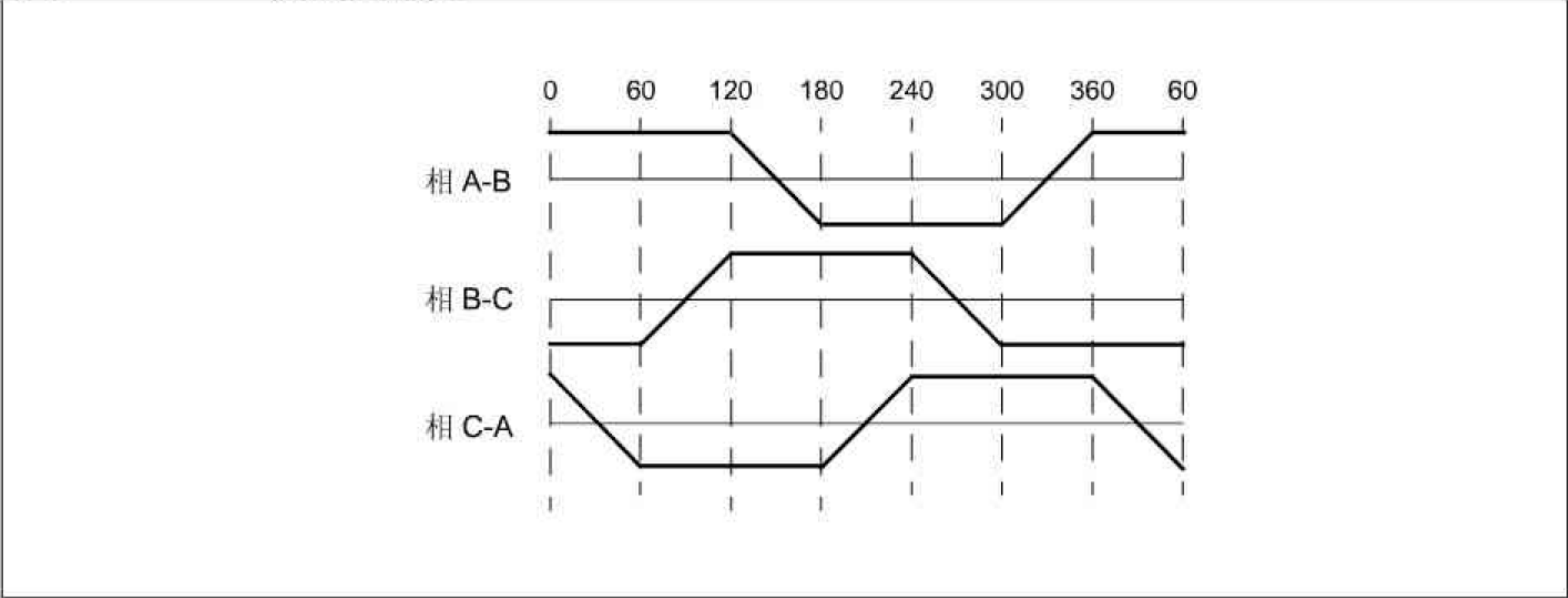
图 1: 梯形反电动势
