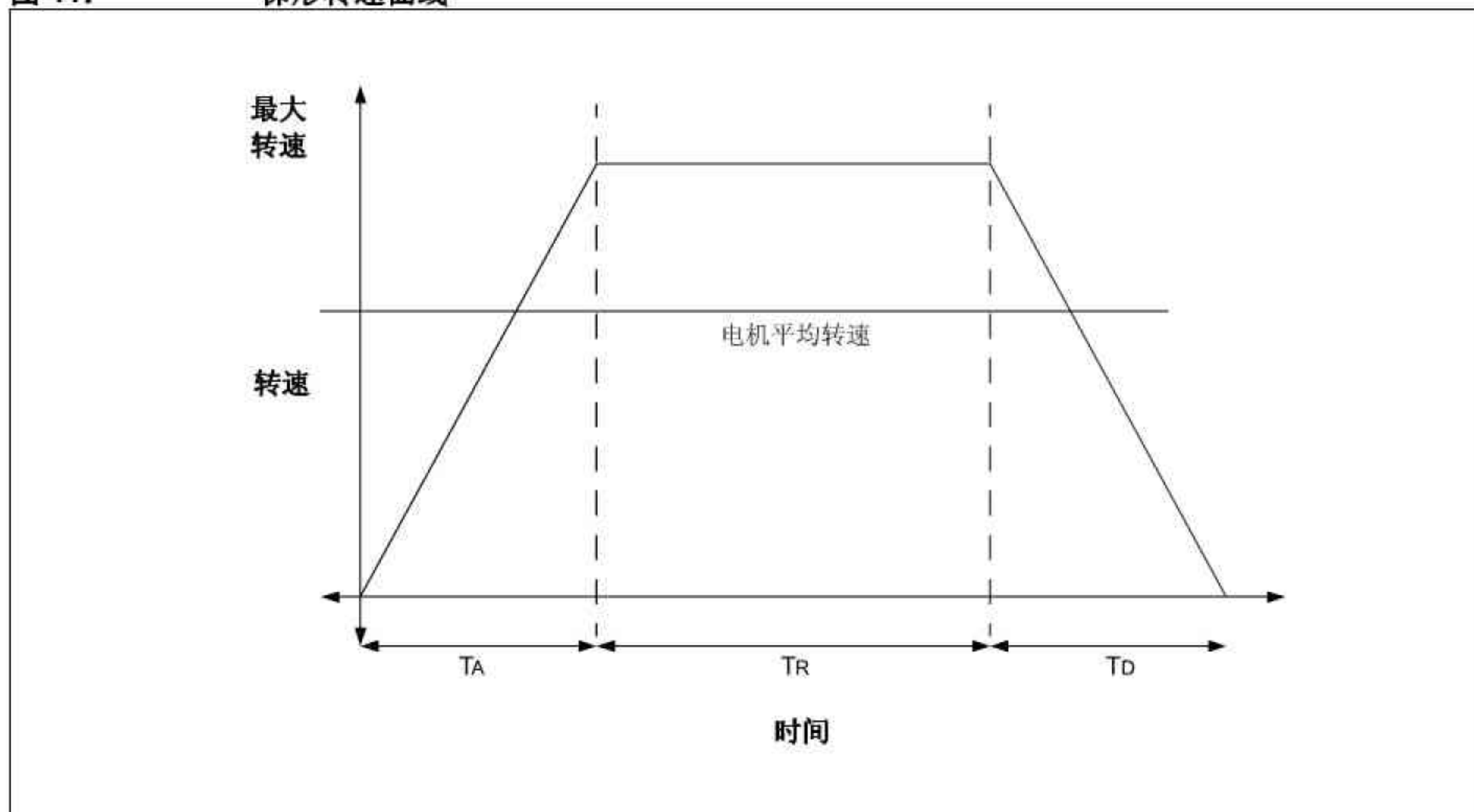
图 11: 梯形转速曲线
