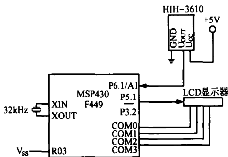
图 1 湿度计电路
